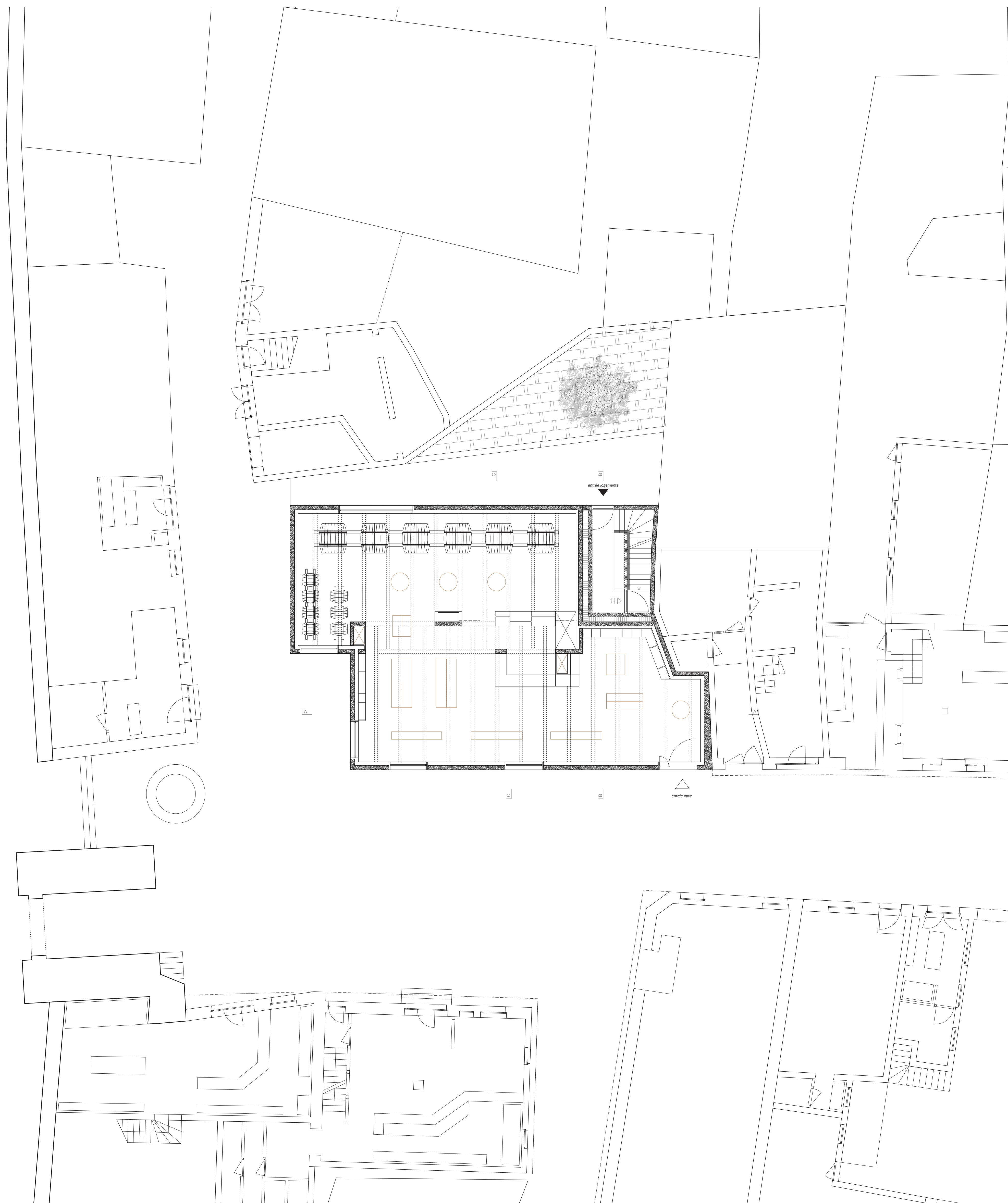
PLAN REZ-DE-CHAUSSÉE
