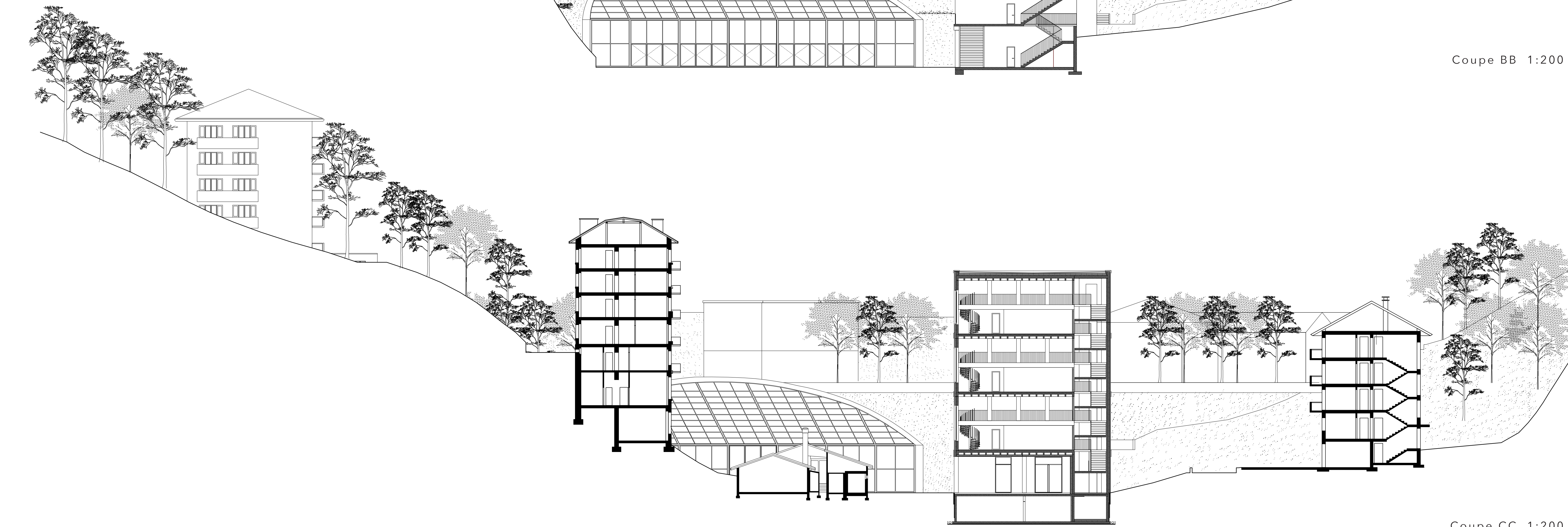
Coupe CC 1:200
