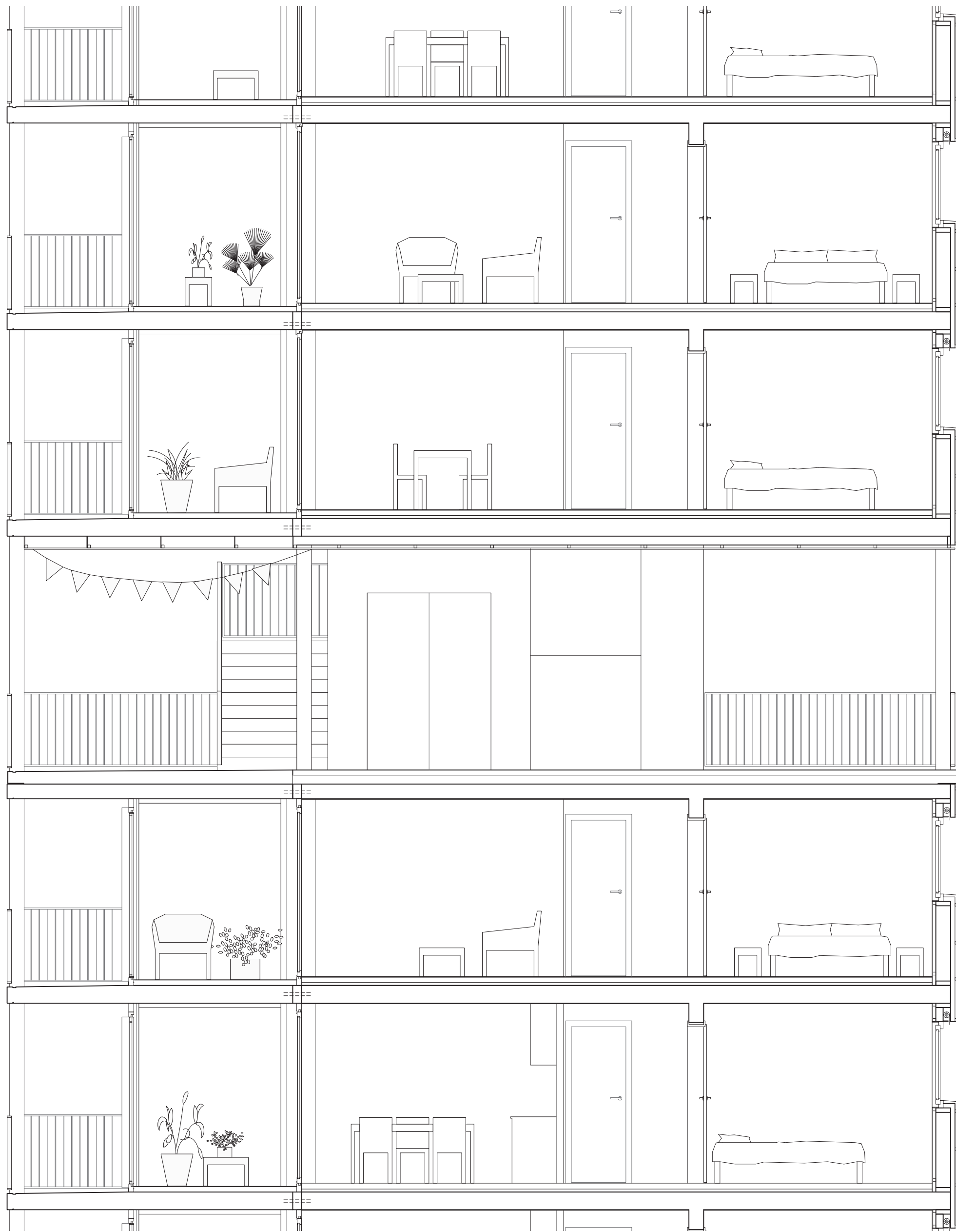
Coupe 1:50
