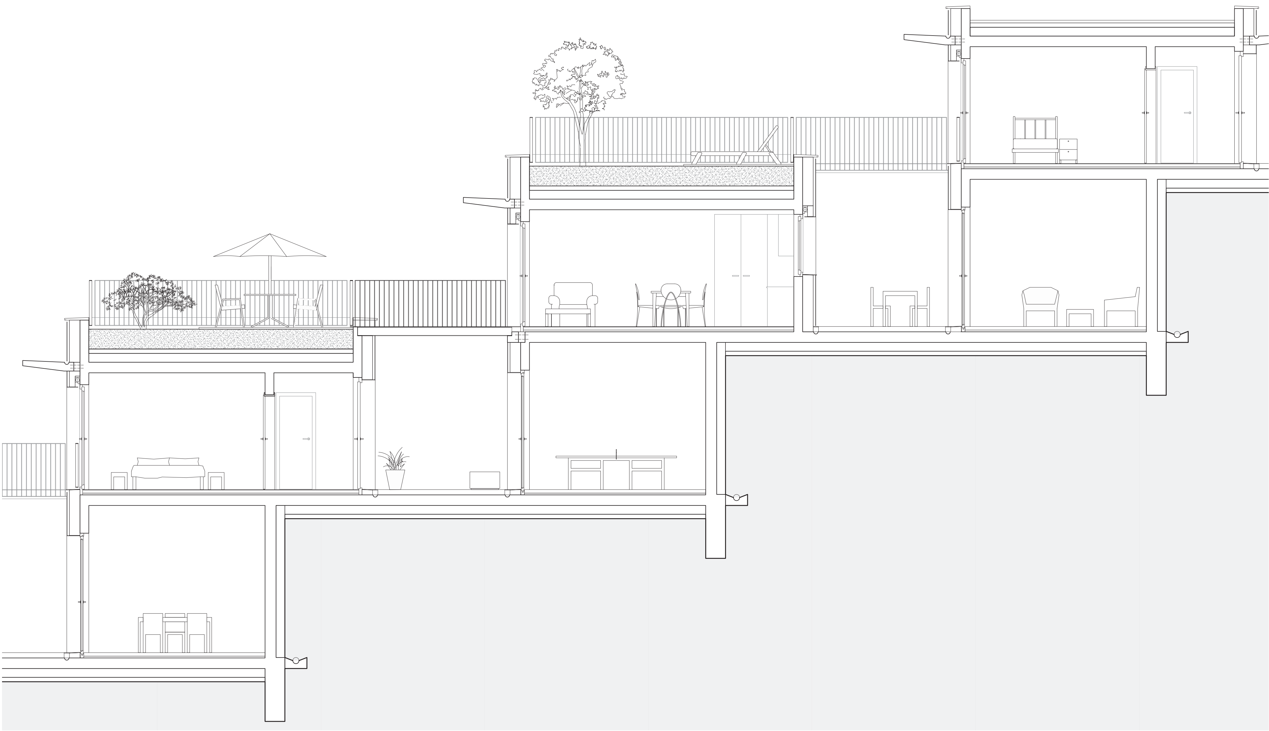
Coupe 1:50
