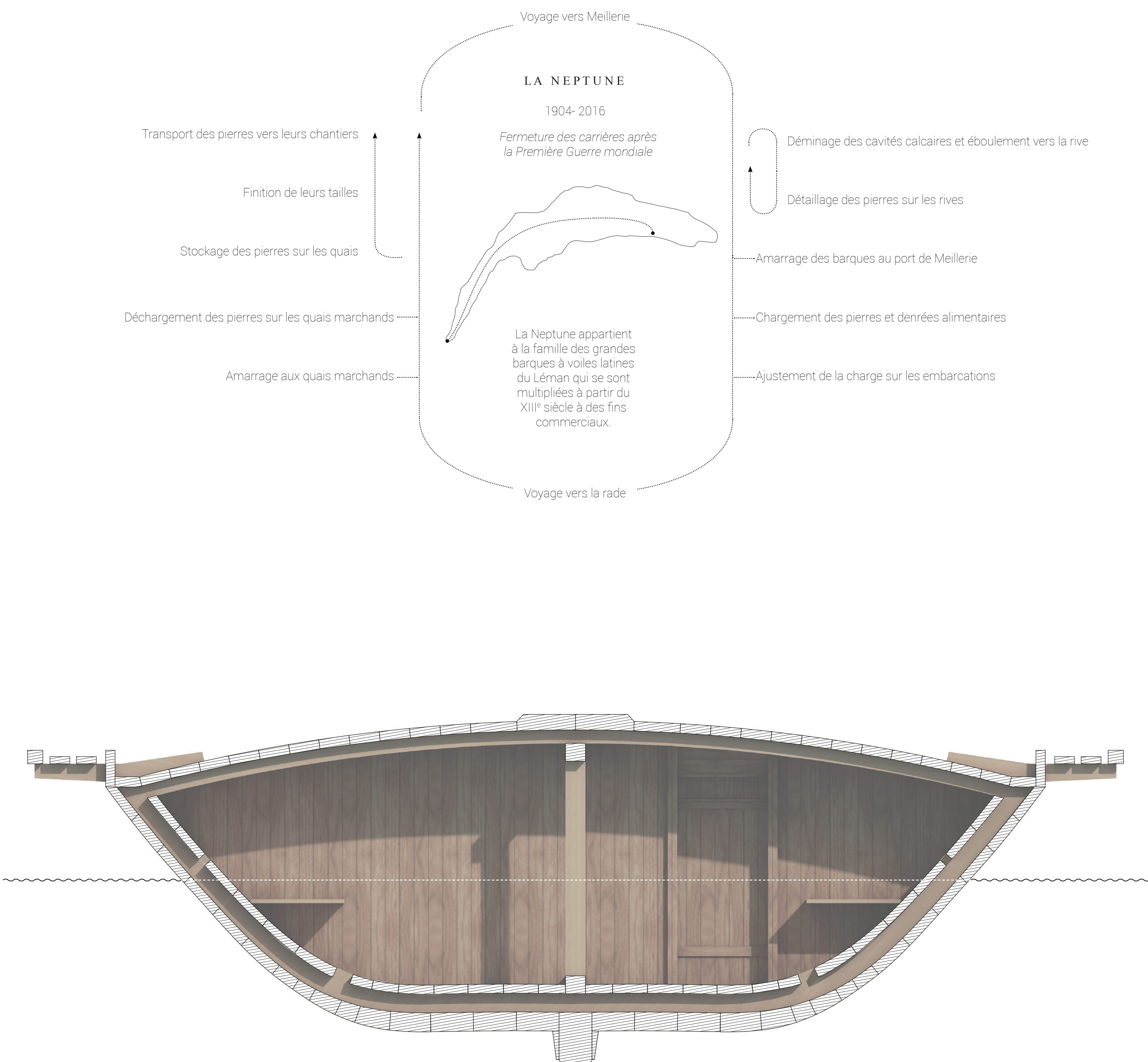
Coupe transversale de la Neptune Échelle : 1/25 e
