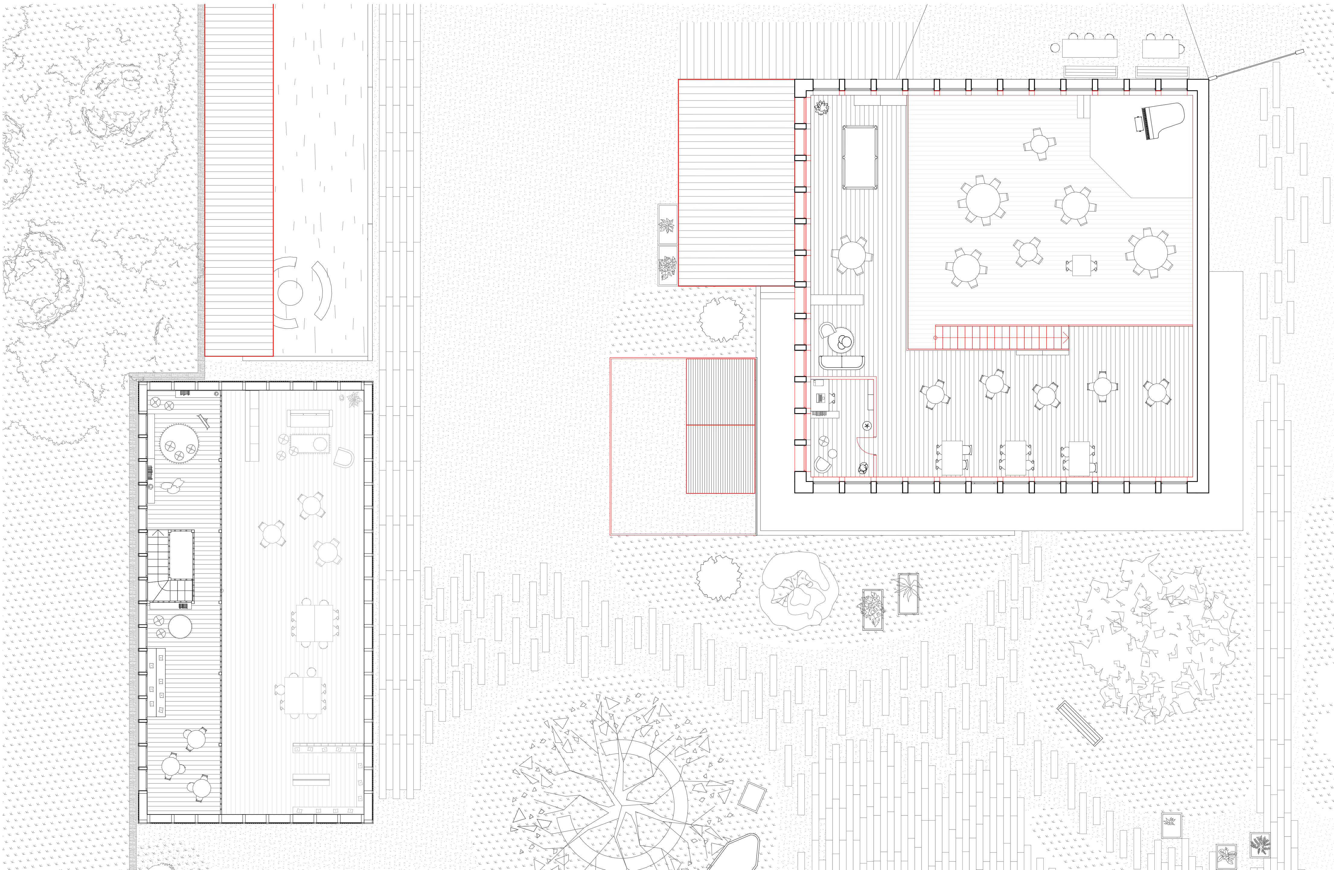
Plan Etage 1:100
