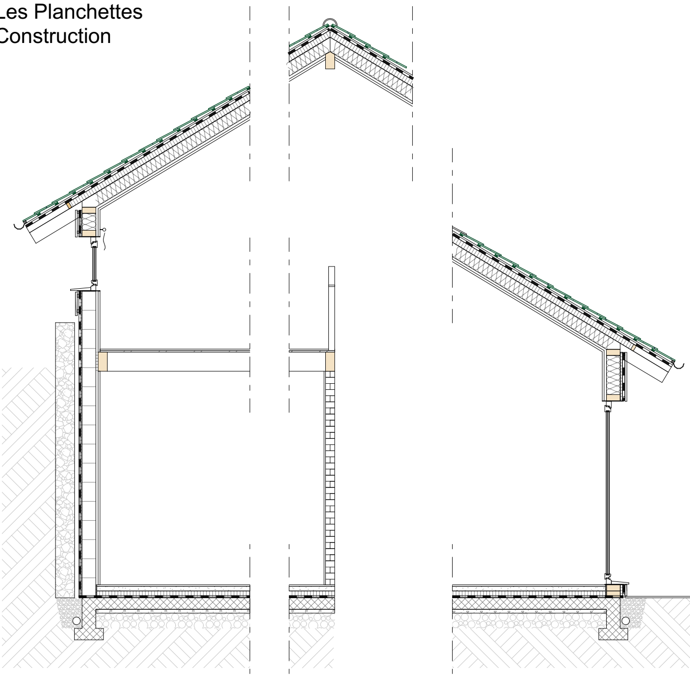
Composition de la toiture
