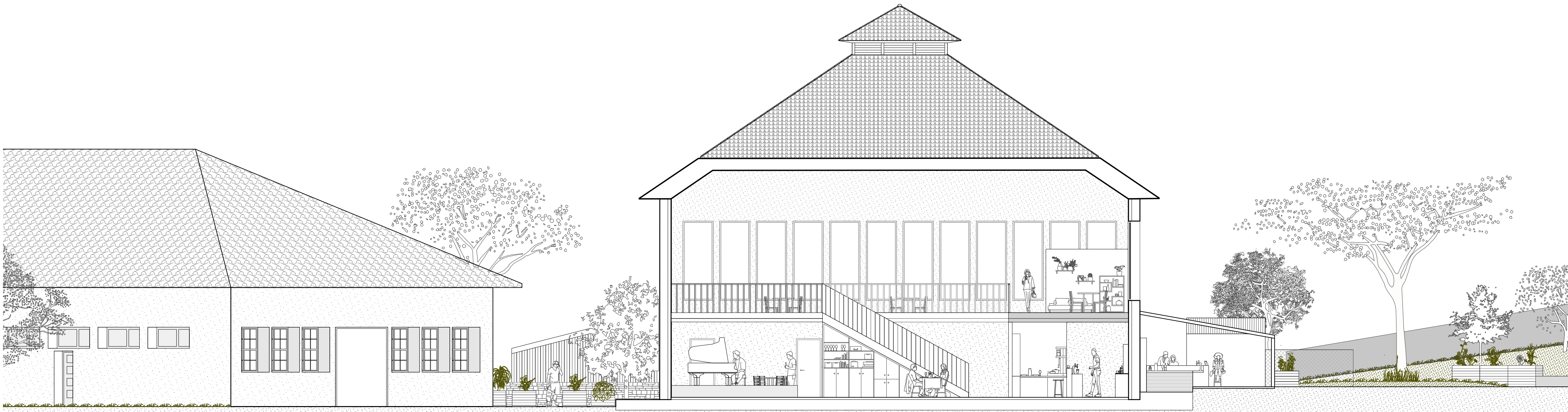
Coupe 1:100
