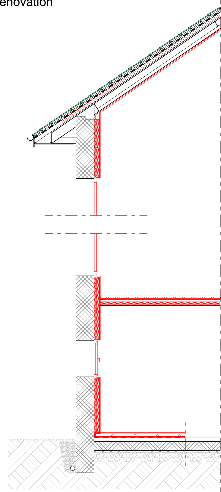
Composition Toiture
