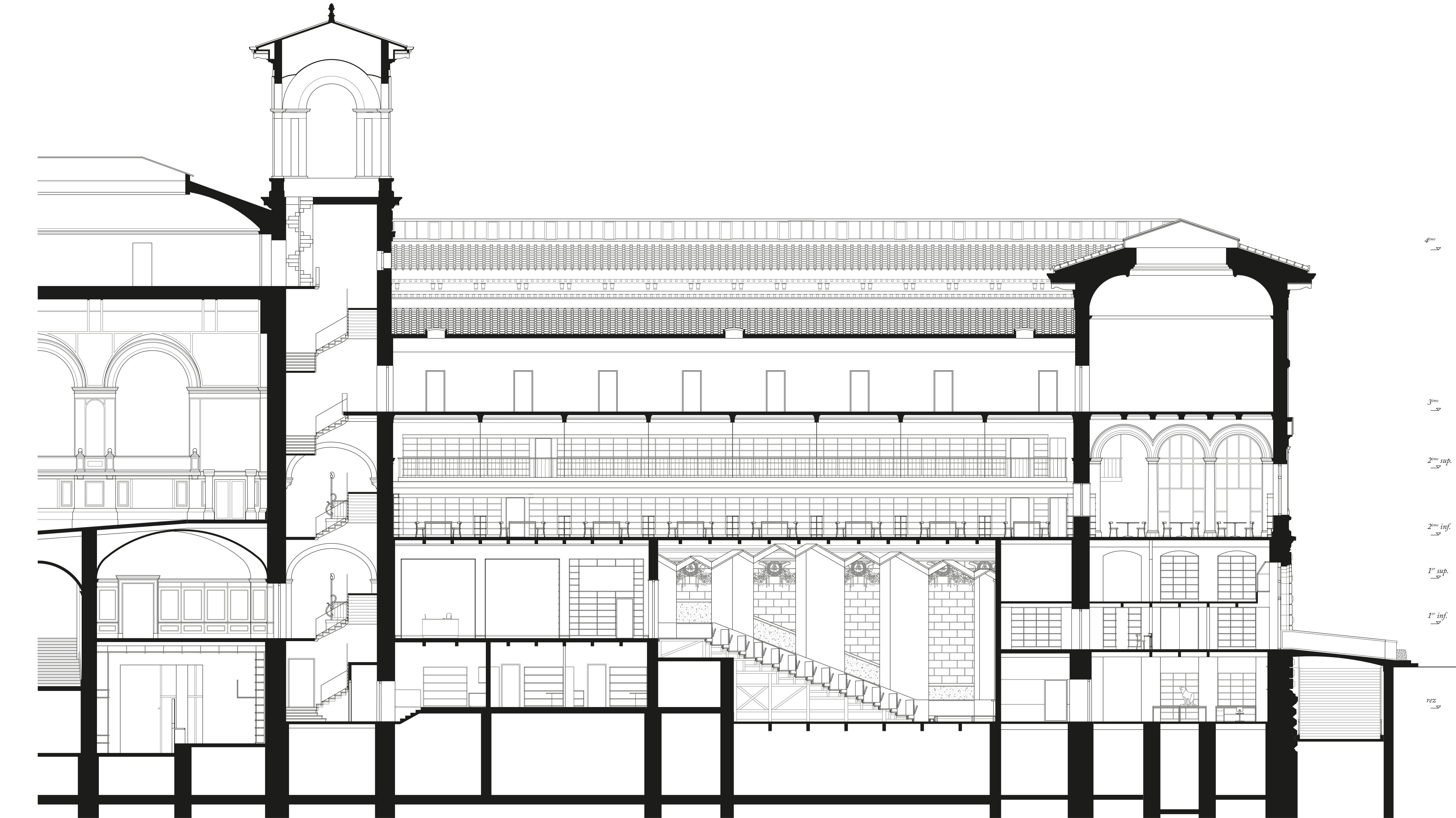
Coupe DD' - 1:150
