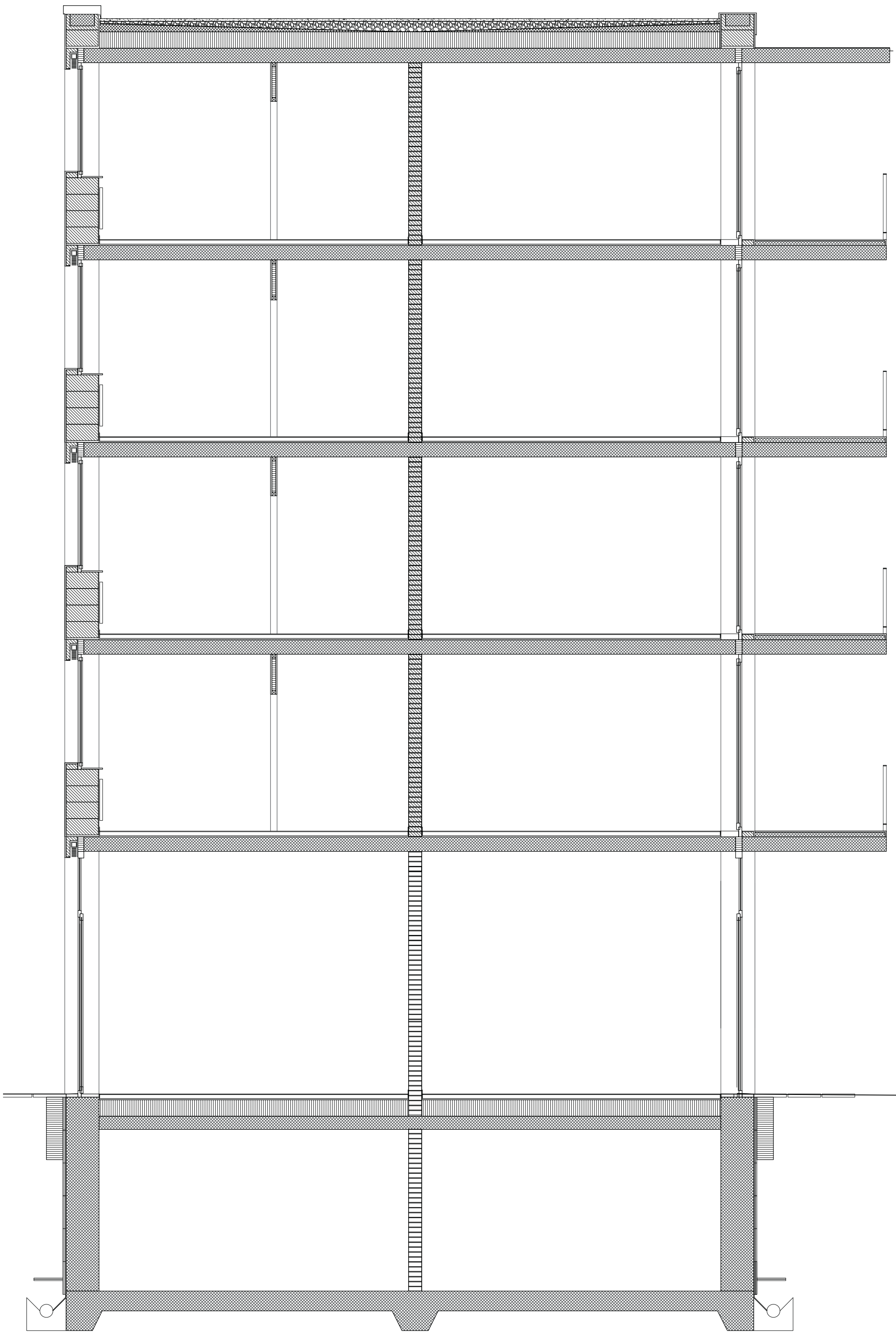
COUPE CONSTRUCTIVE 1:50
