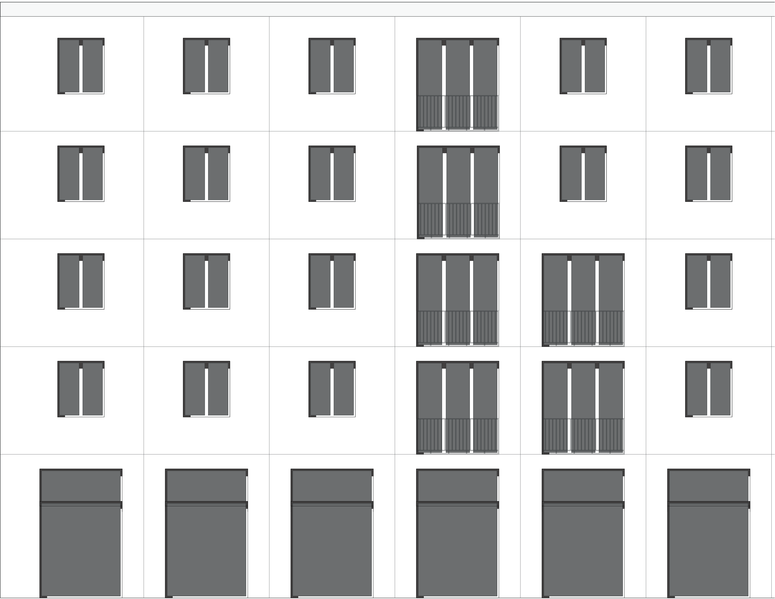
FAÇADE 1:50
