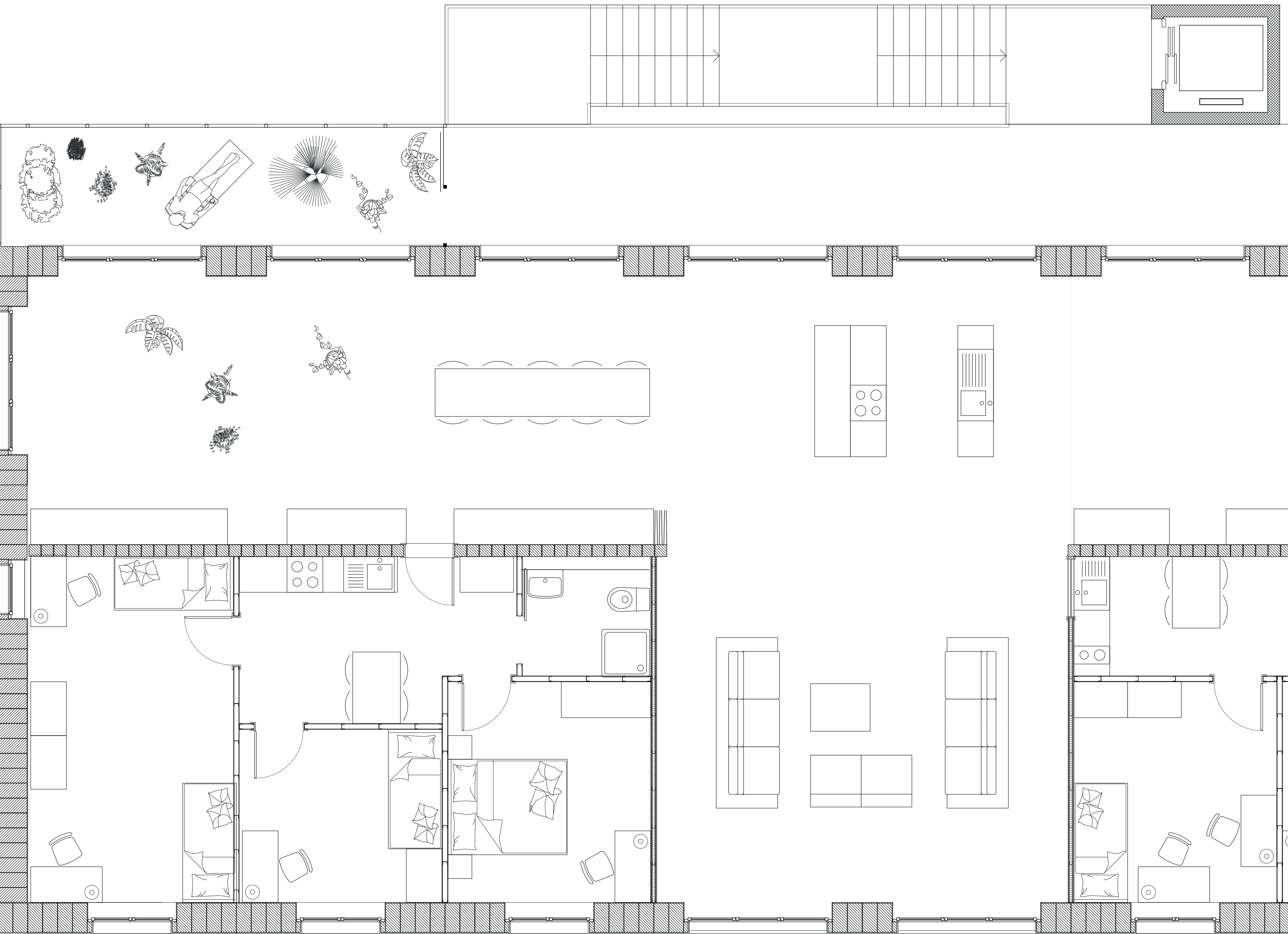
PLAN 1:50
