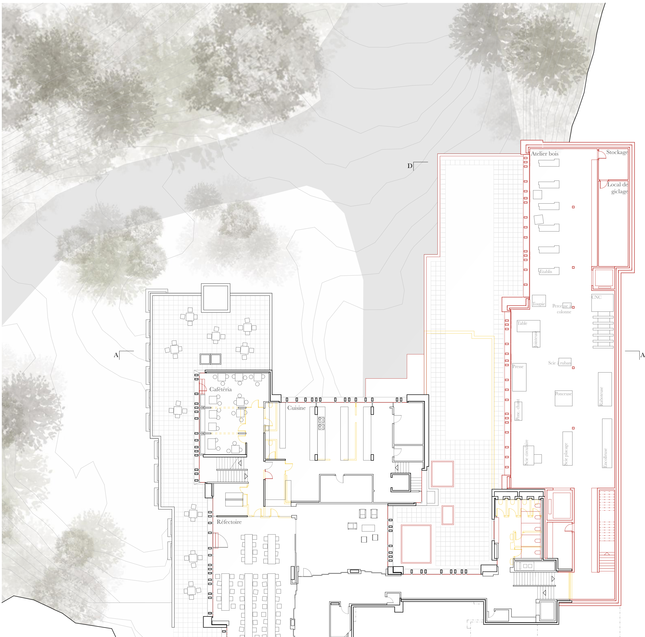
1er sous-sol 1/200
