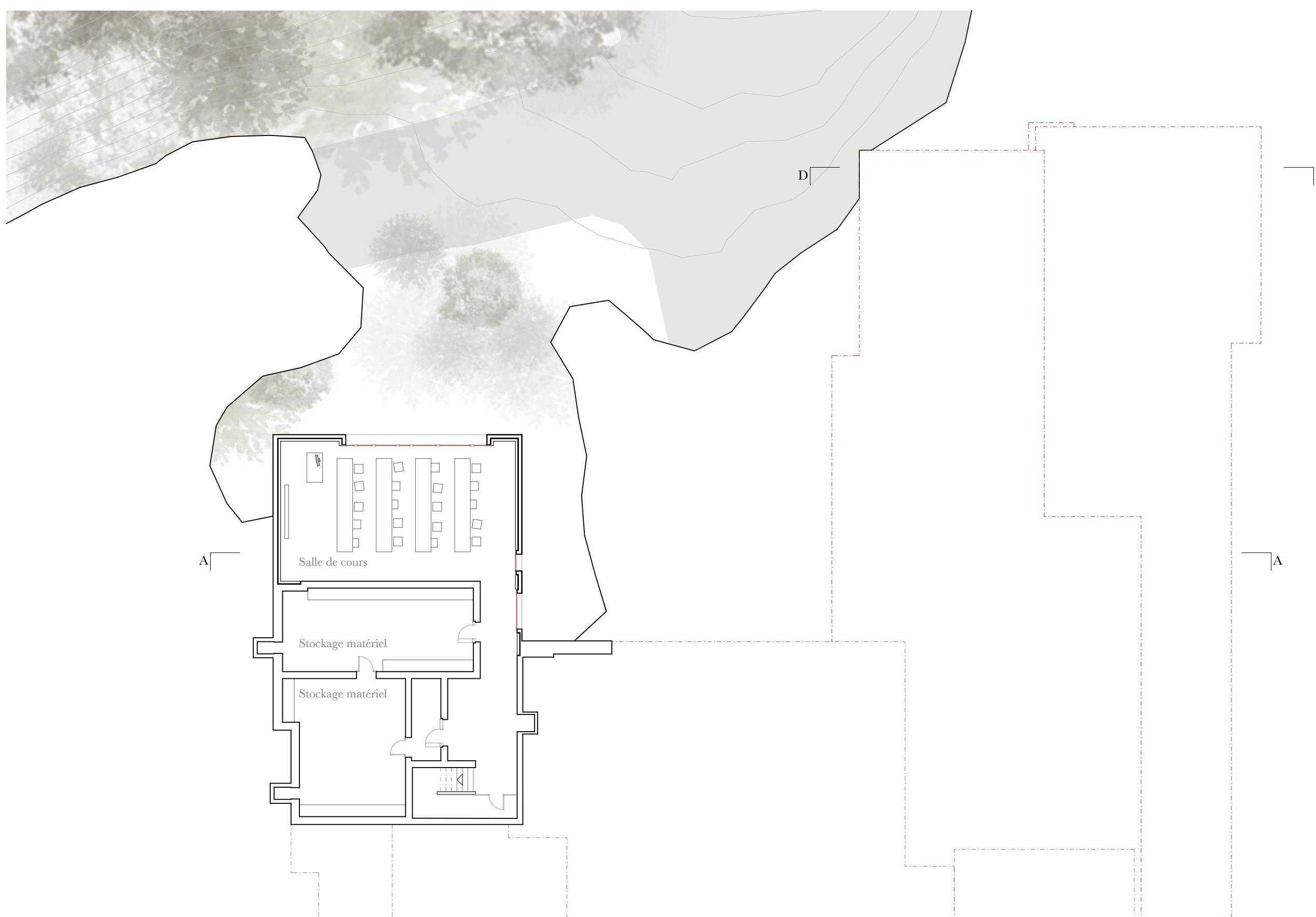
3ème sous-sol 1/200
