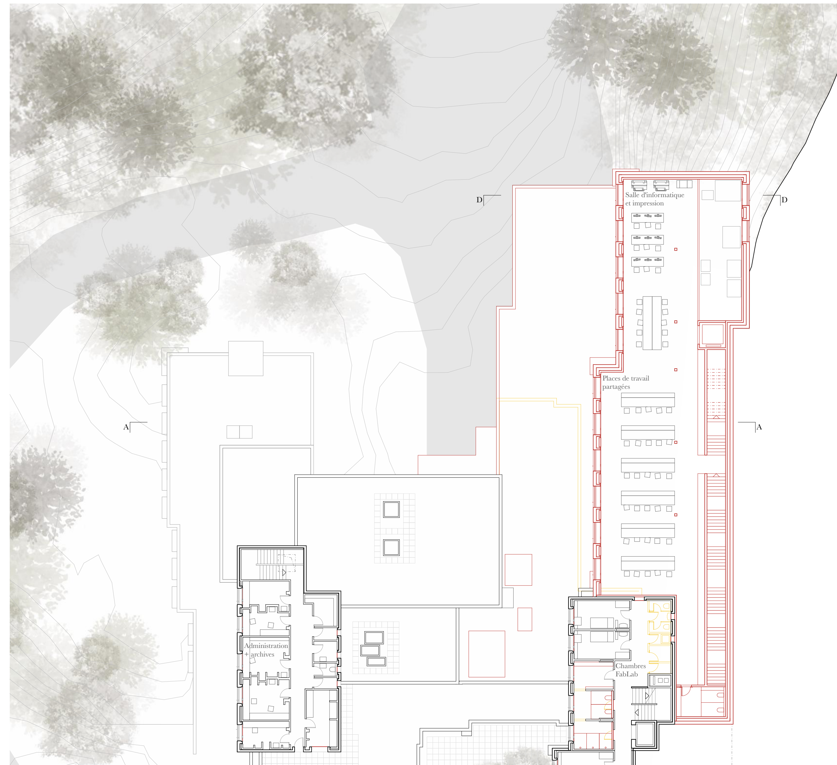
1er étage 1/200
