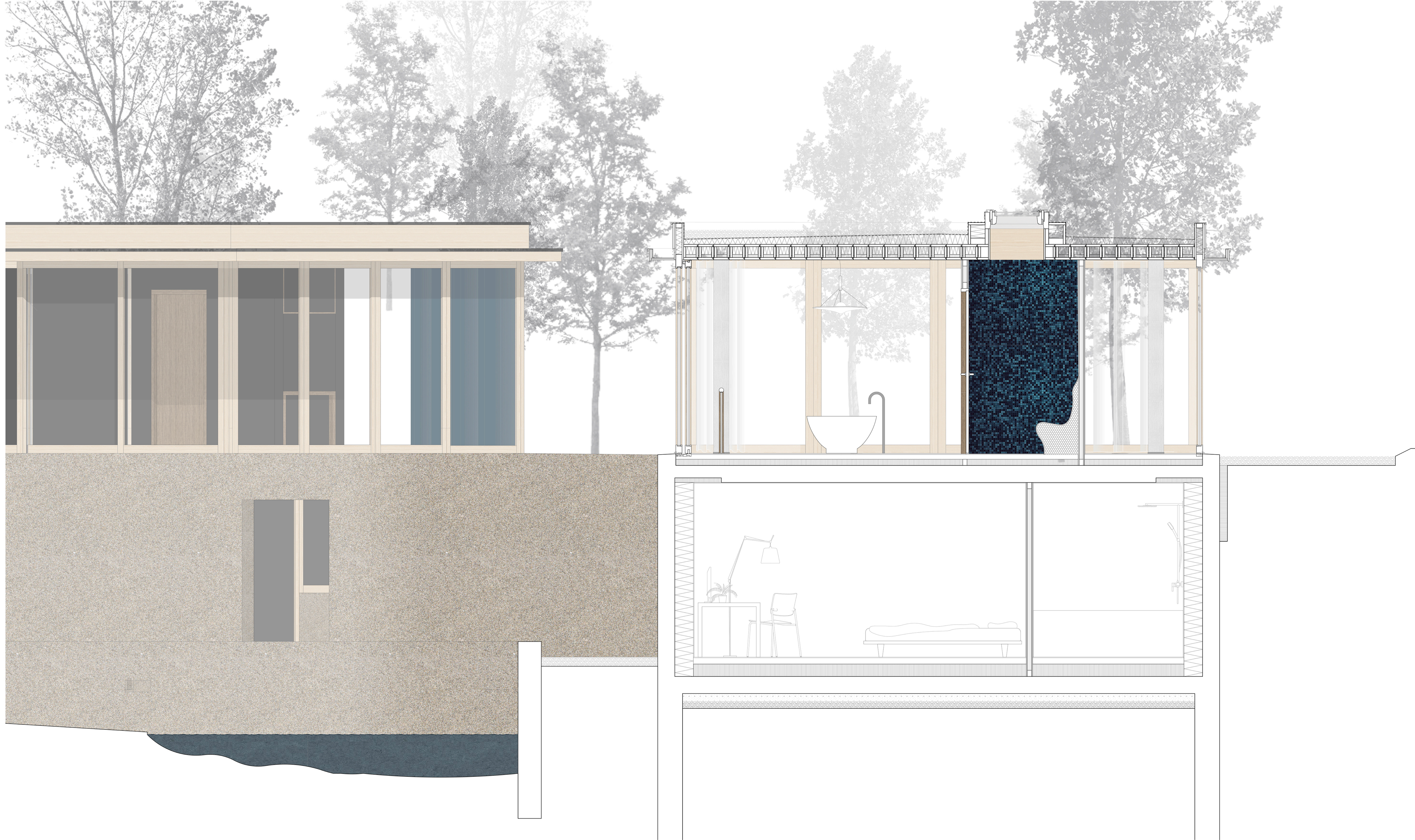
Pavillon de naissance - coupe transversale constructive - 1/20
