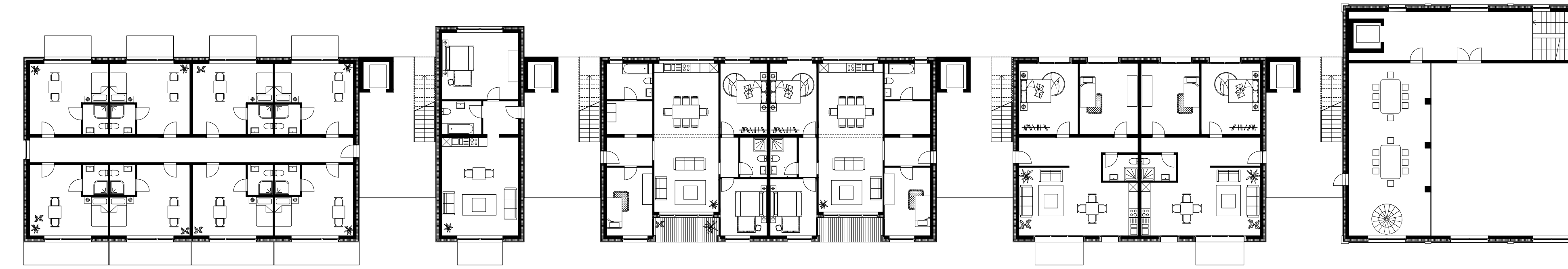
Etage type (sauf mezzanine de la maison de quartier) 1:200
