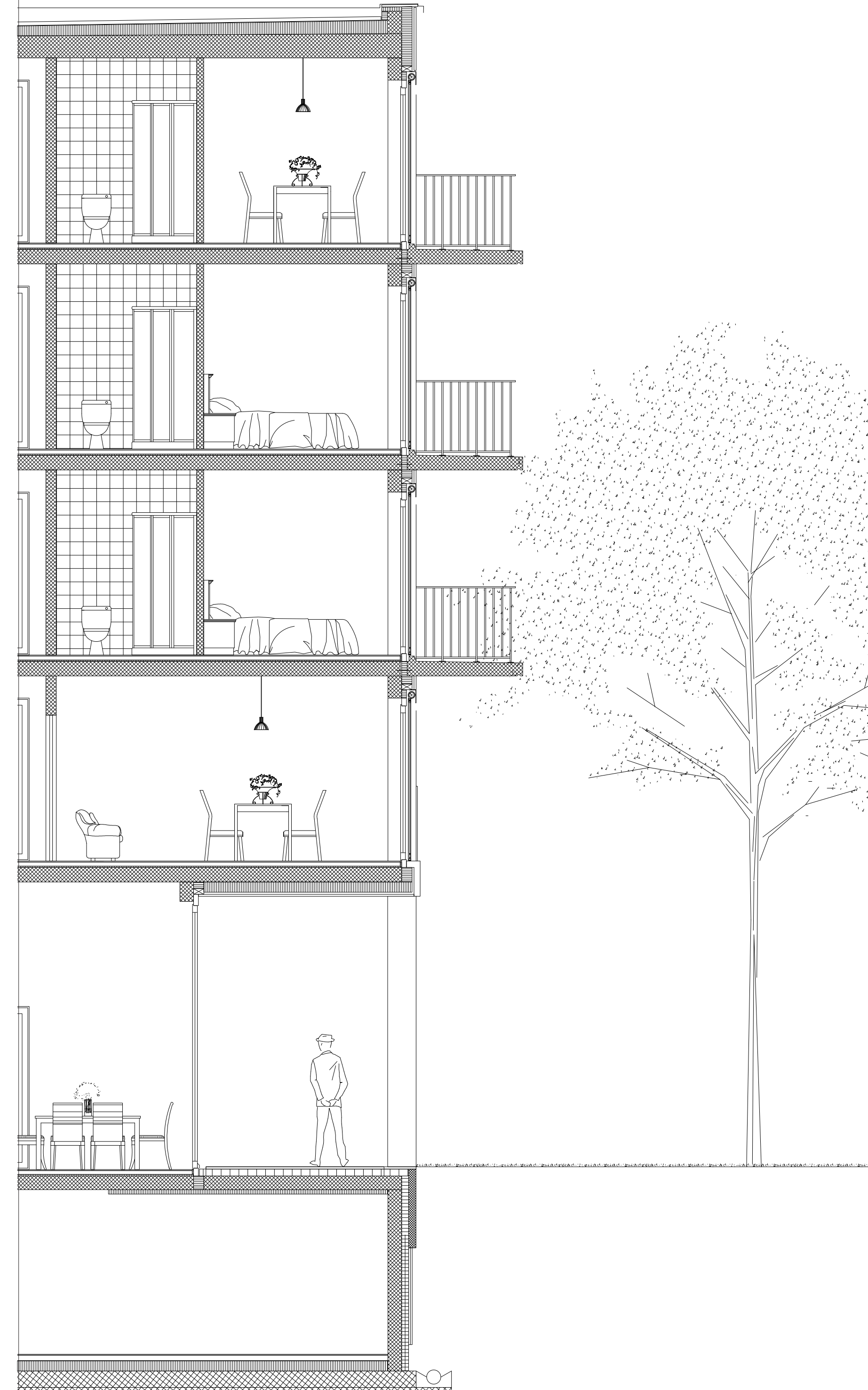
Details, Logements sociaux, 1:50
