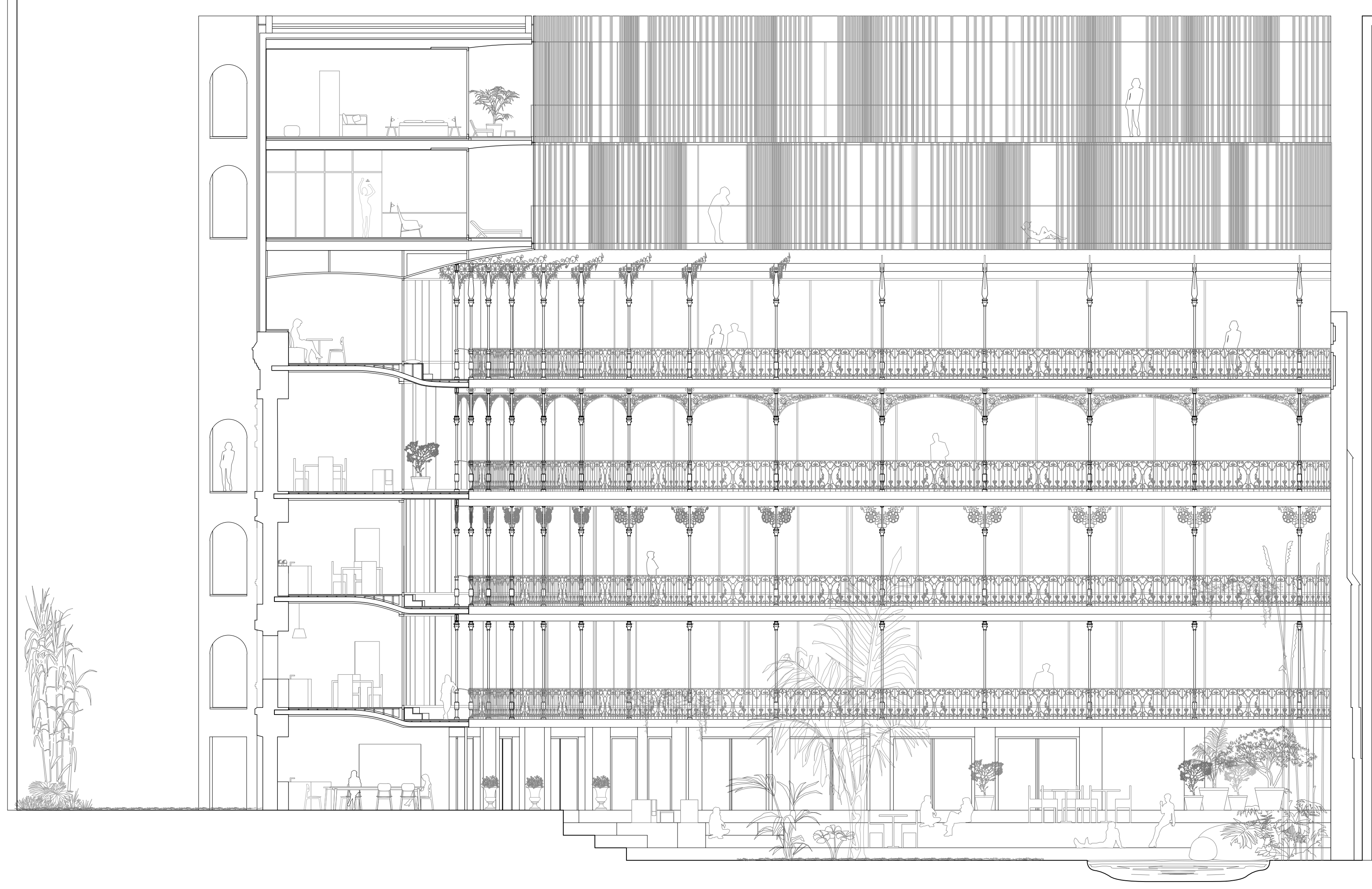
Coupe aa'
