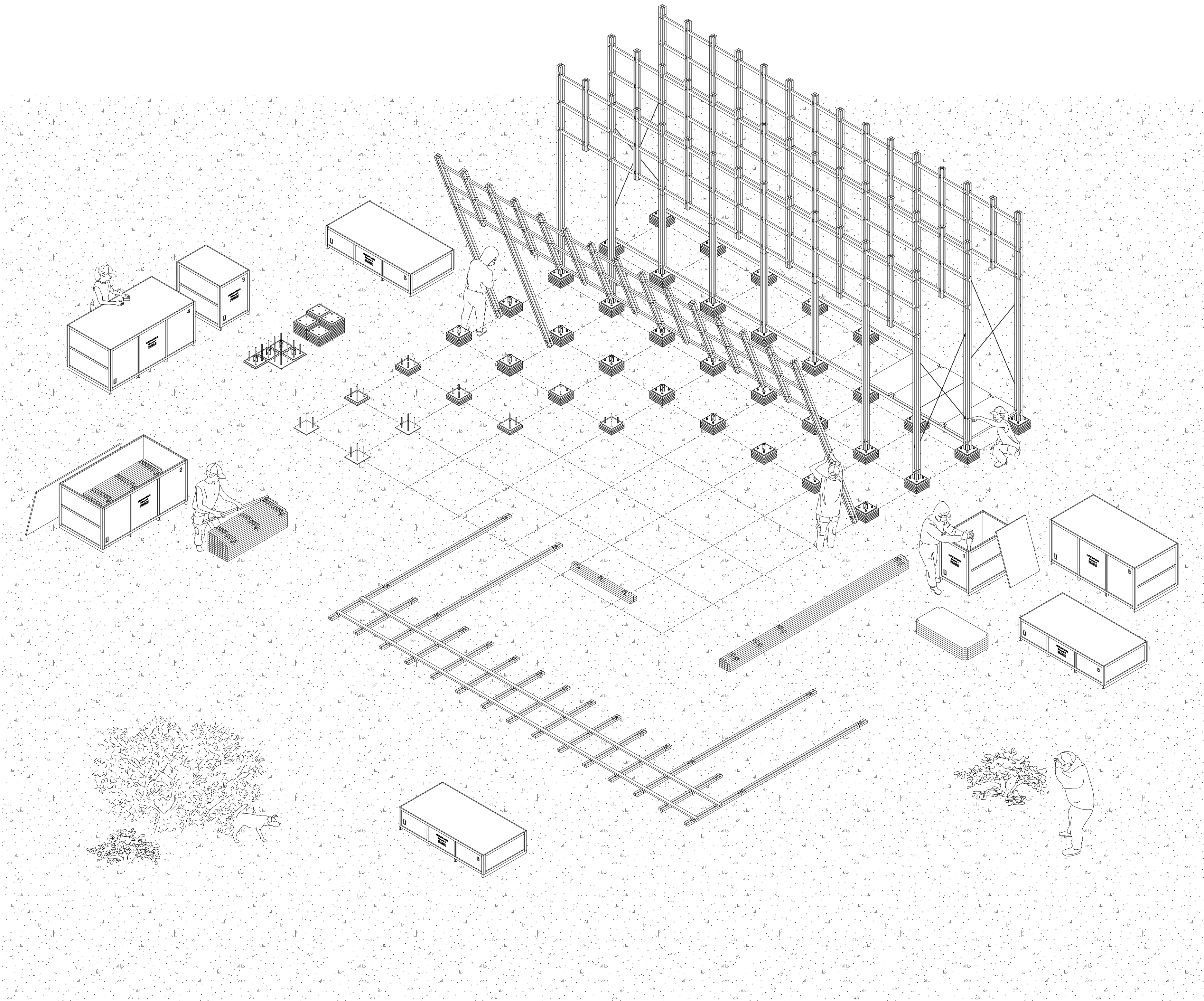
Isométrie montage 1:50
