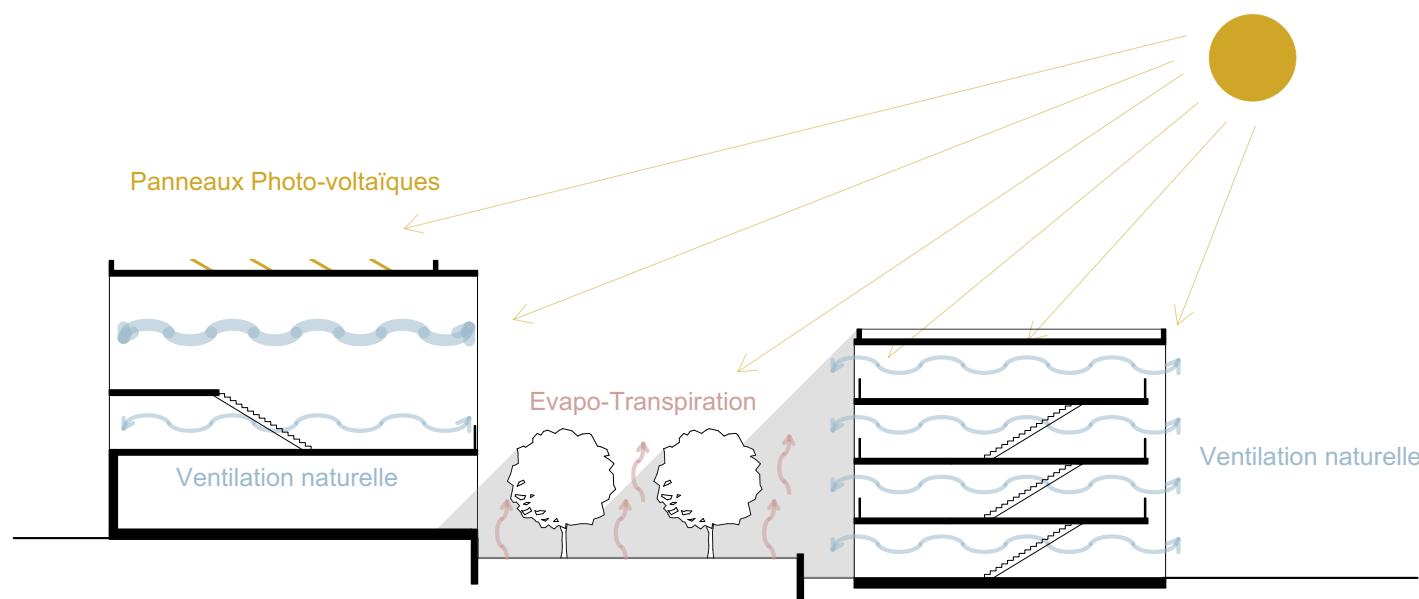
Schéma du concept bioclimatique
