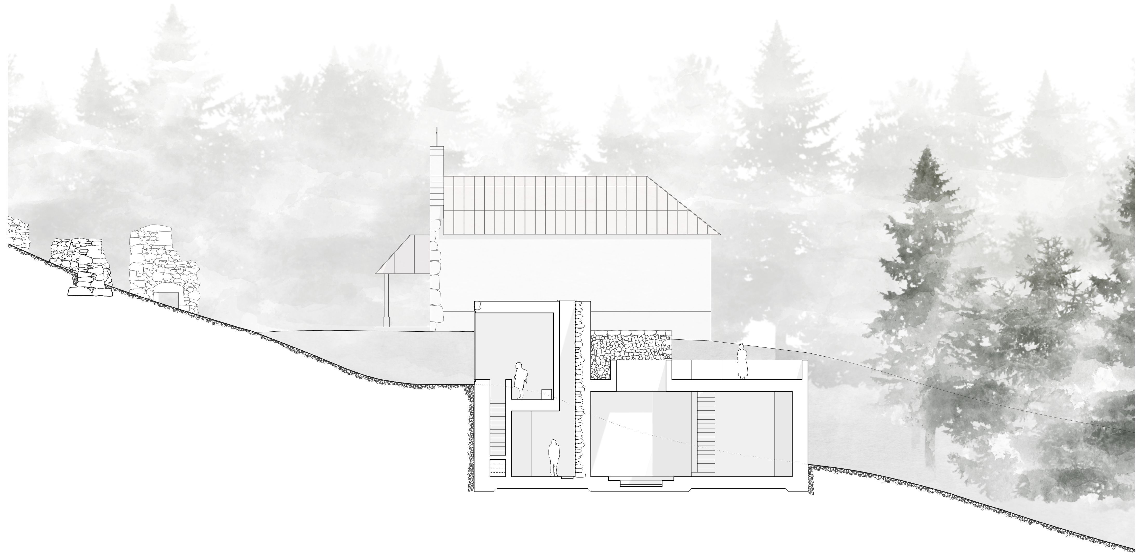
COUPE BB SUD EST / NORD OUEST
