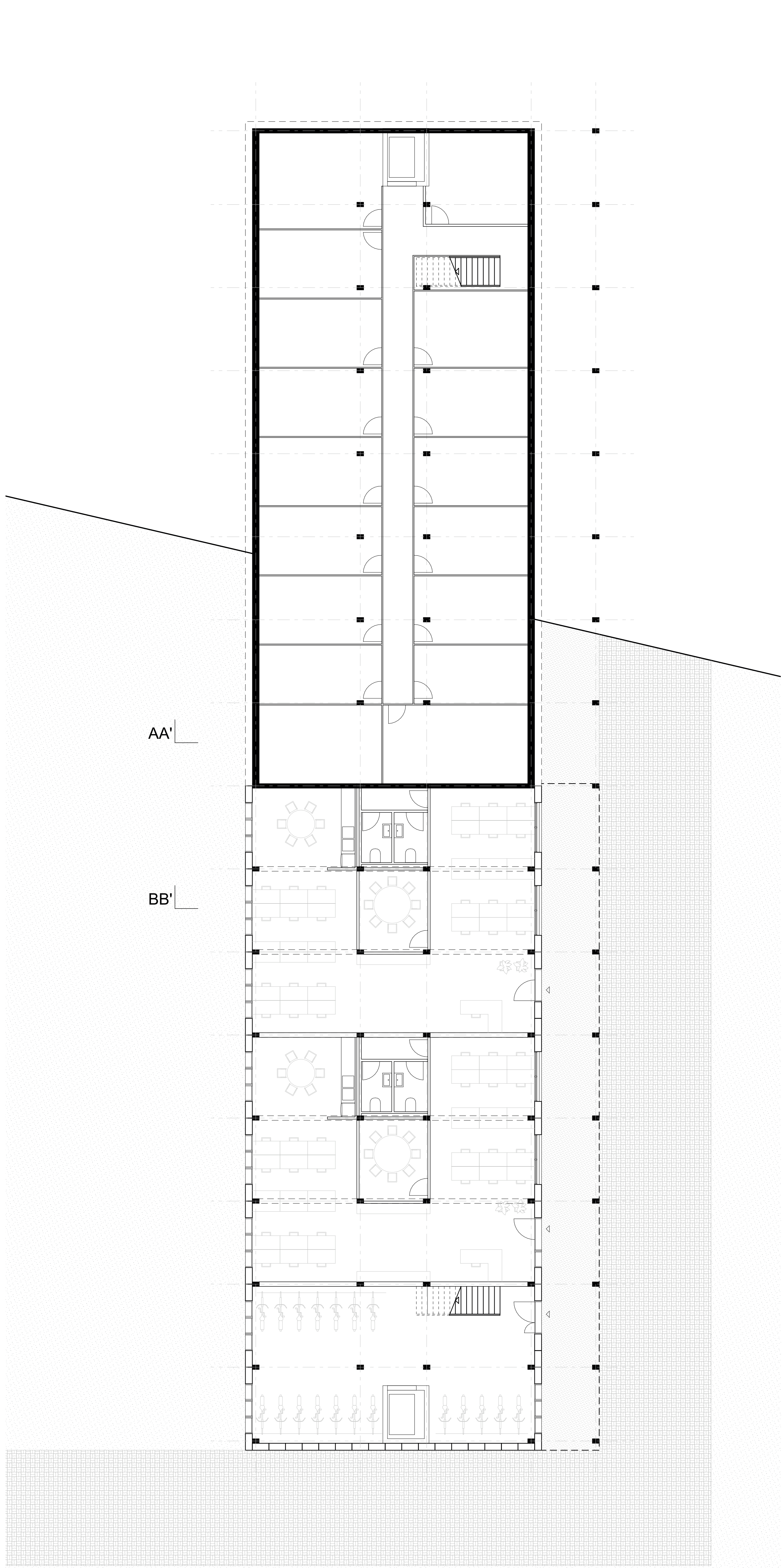
⊙ Plan rez inférieur 1:100
