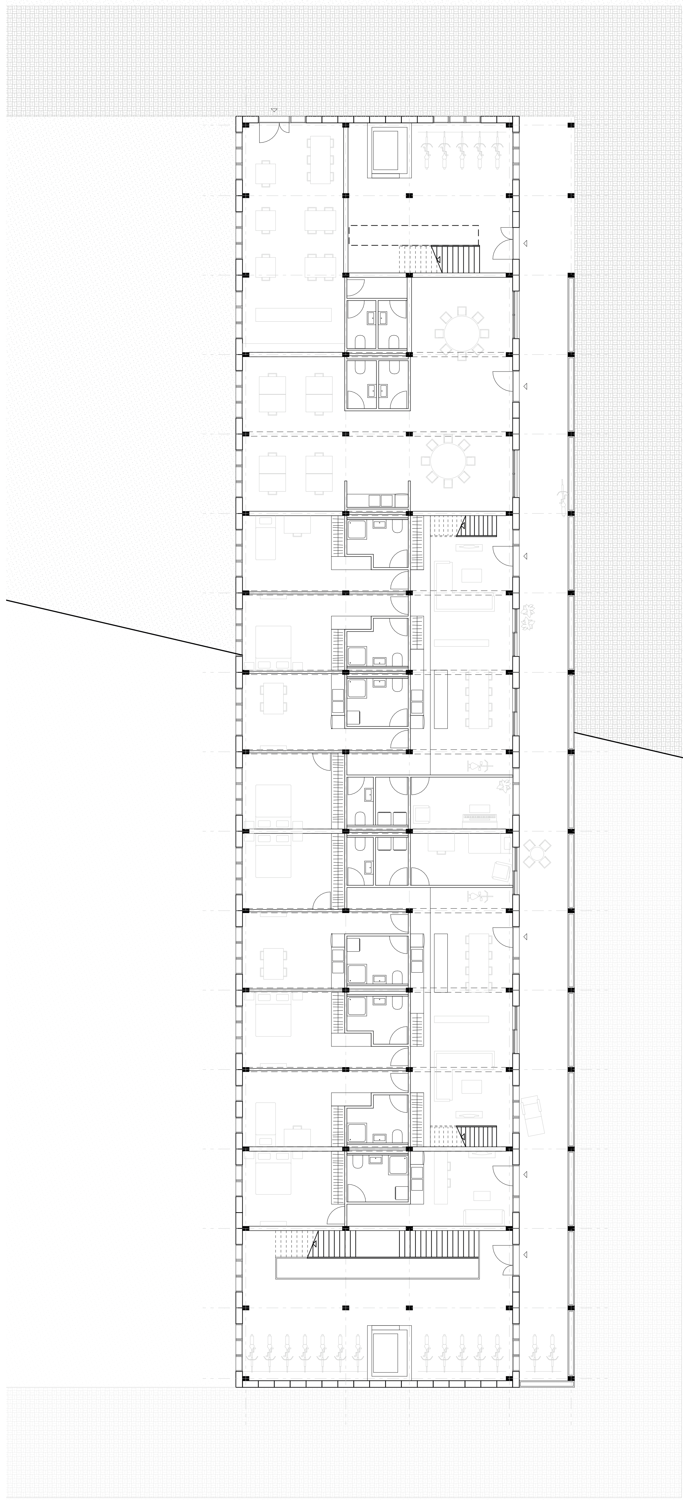
⊙ Plan rez supérieur 1:100
