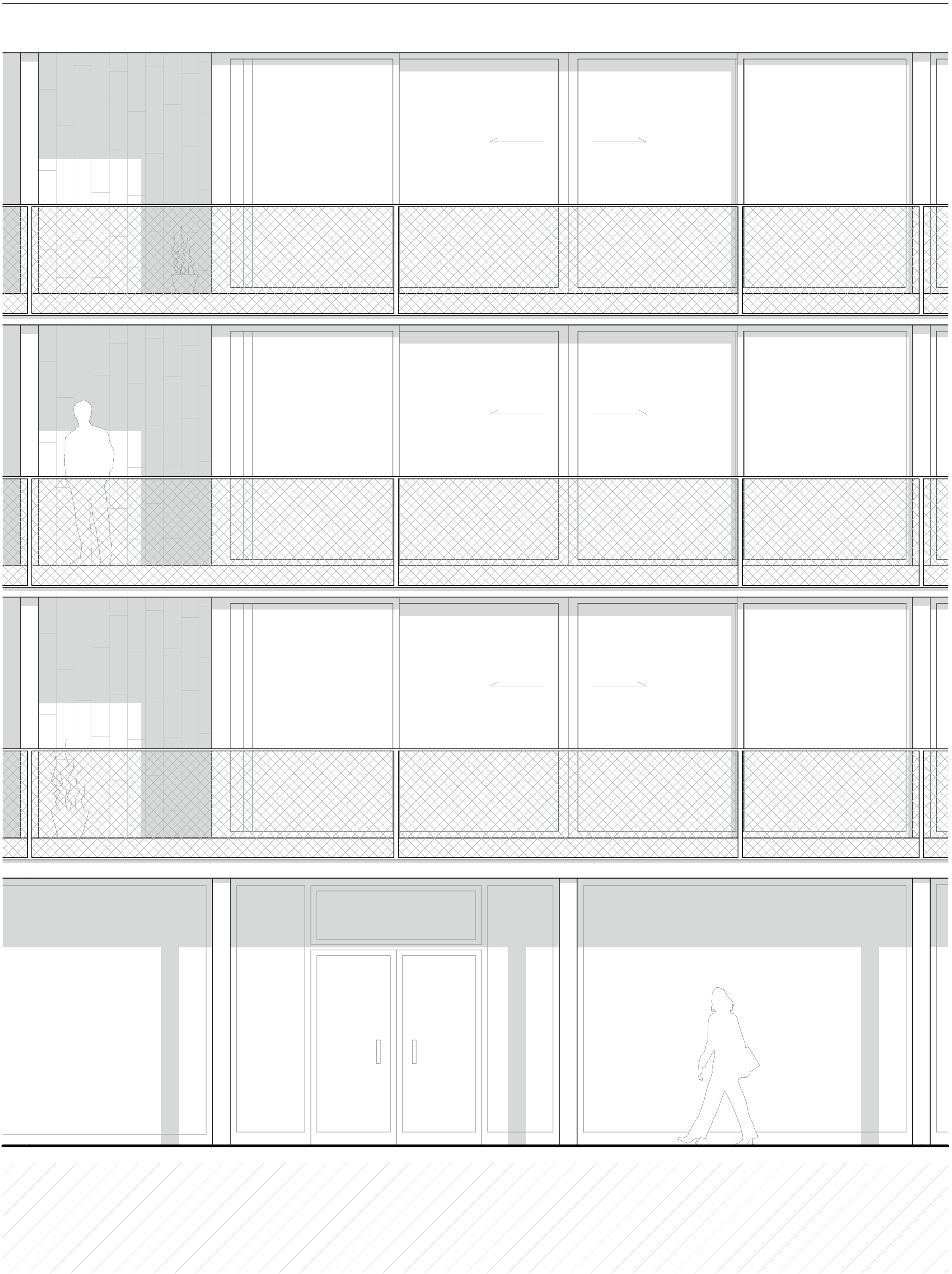
Détails constructifs façade Nord 1 : 33
