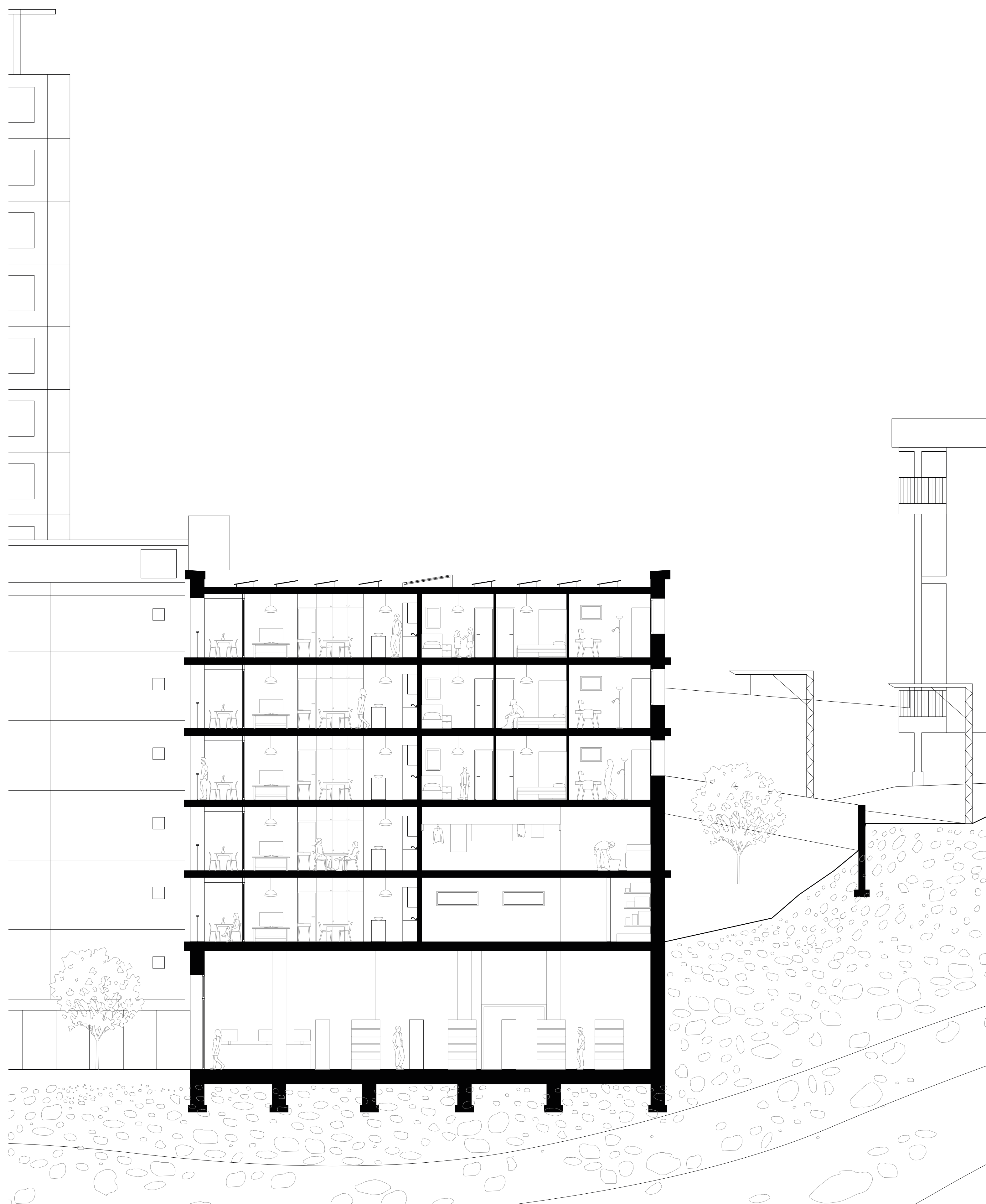
Coupe Transversale 1:100
