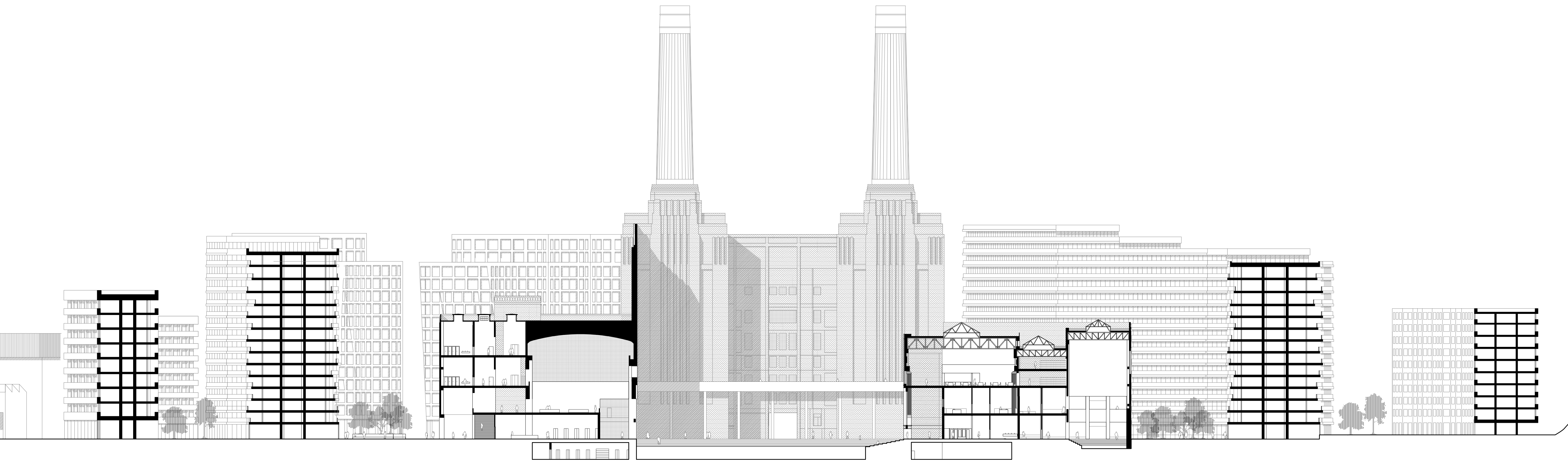
Section A-A' 1 : 500
