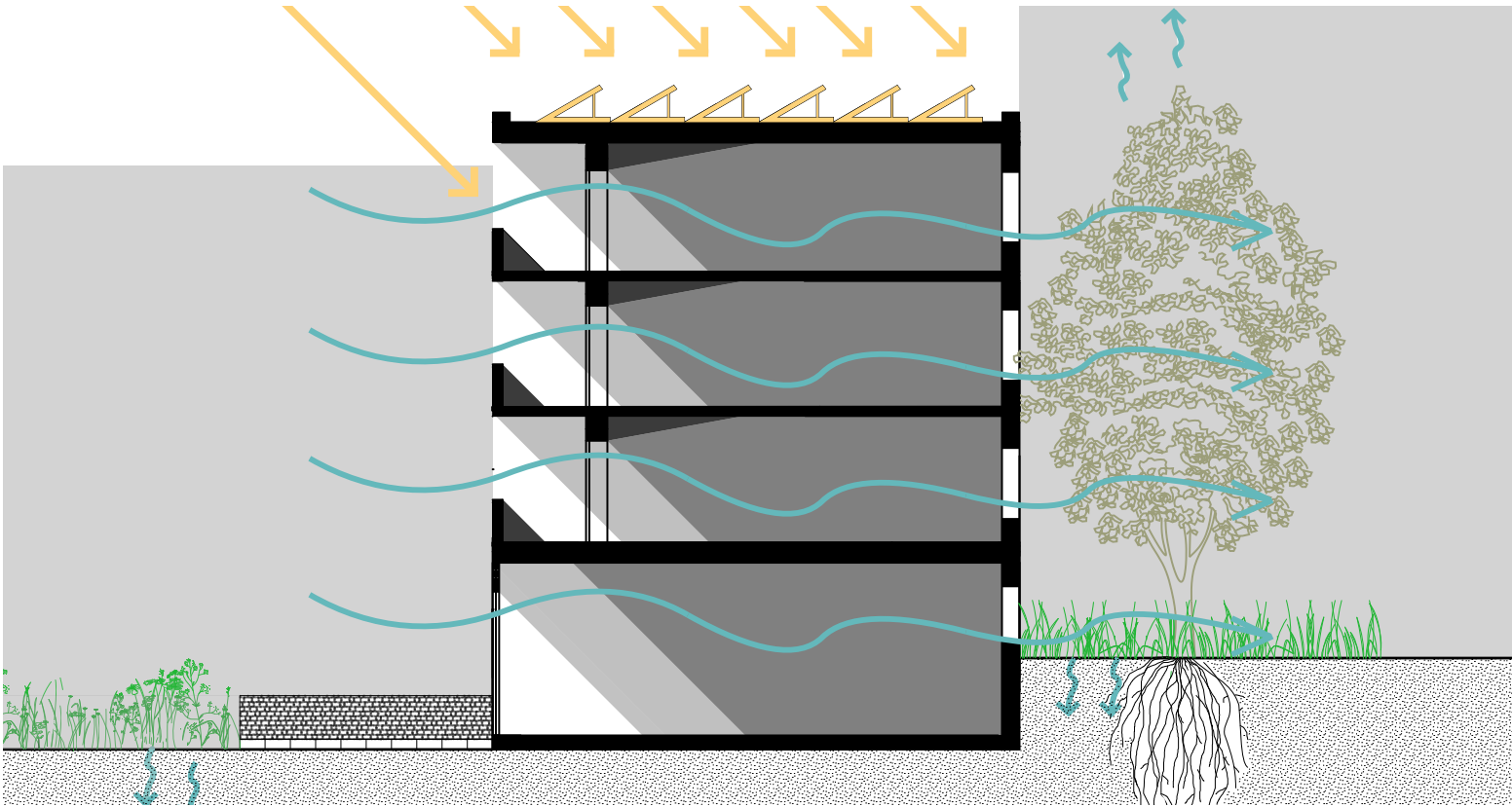
Schéma du concept bioclimatique
