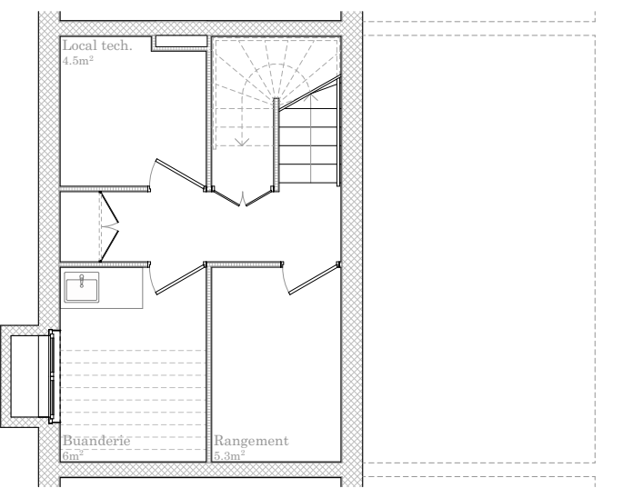
Sous-sol
