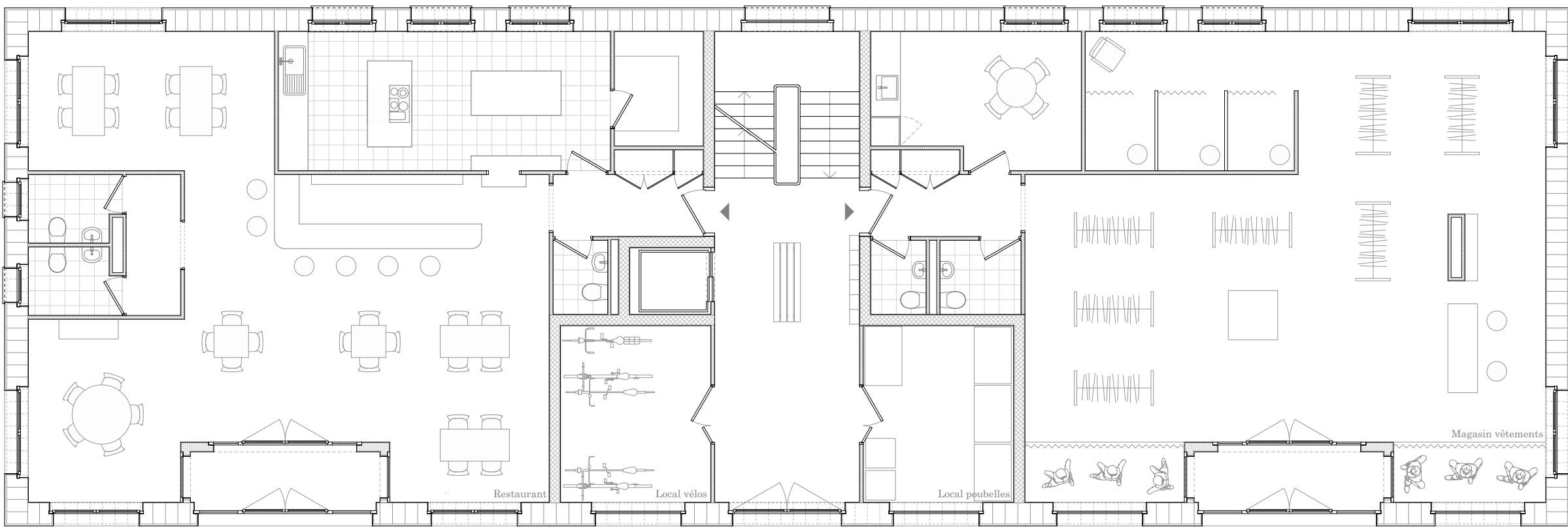
Rez-de-chaussée
