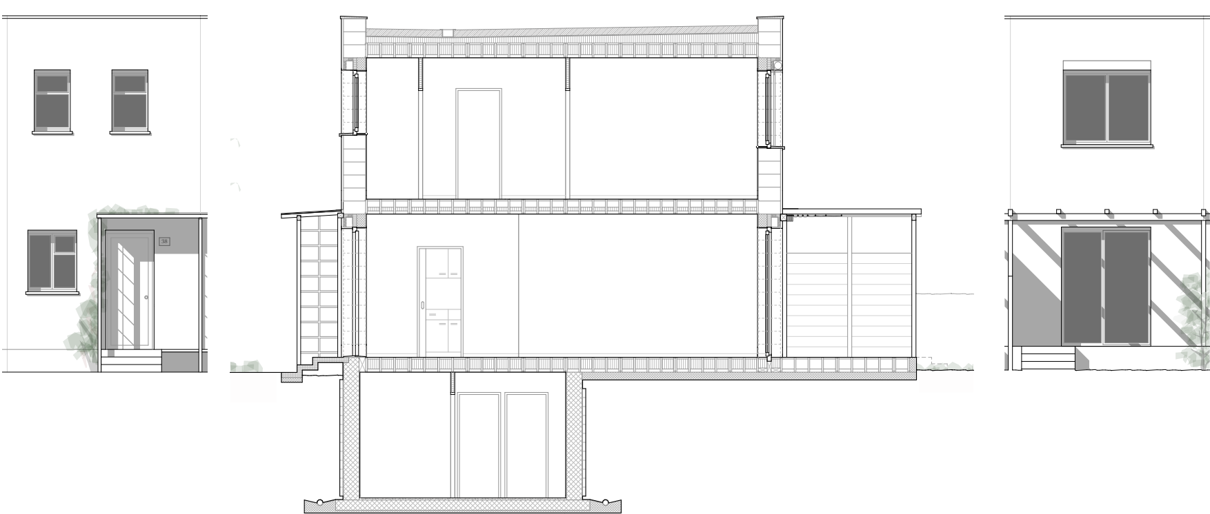
Coupes transversales Façades sur rue et sur jardin 1:100
