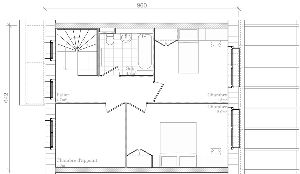
1er étage
