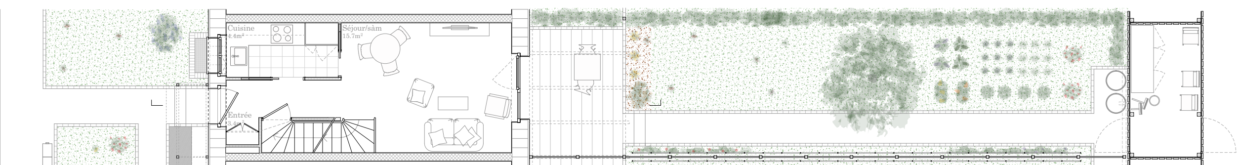
Rez-de-chaussée
