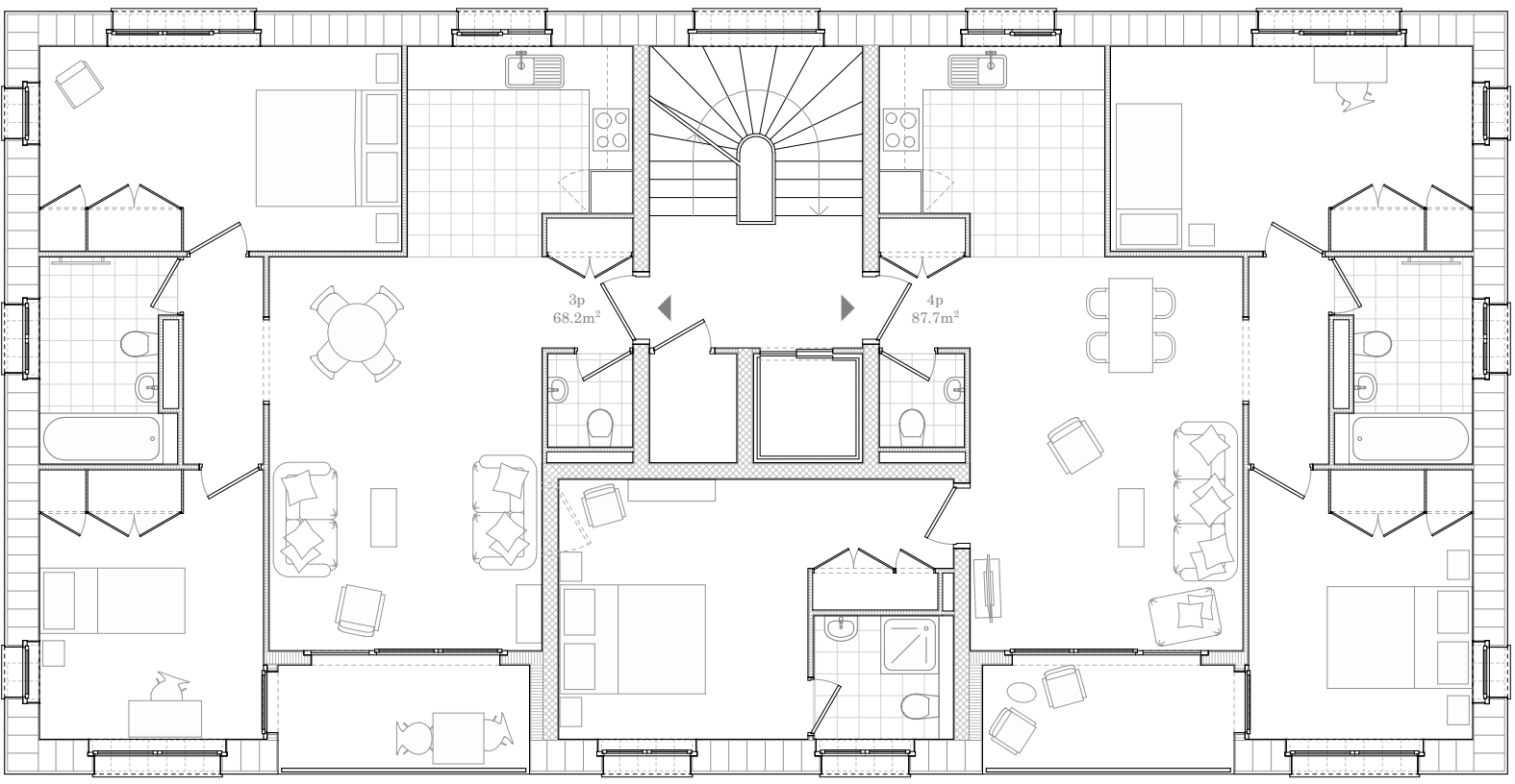
Étage type - Variante 2
