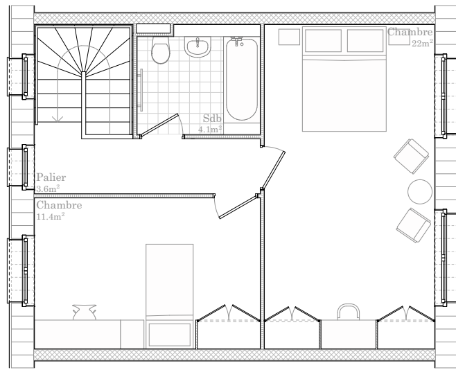
2e étage - Variante 2
