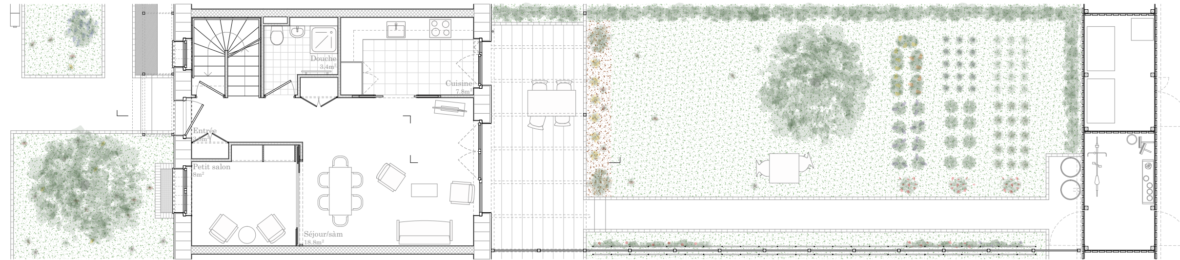
Rez-de-chaussée
