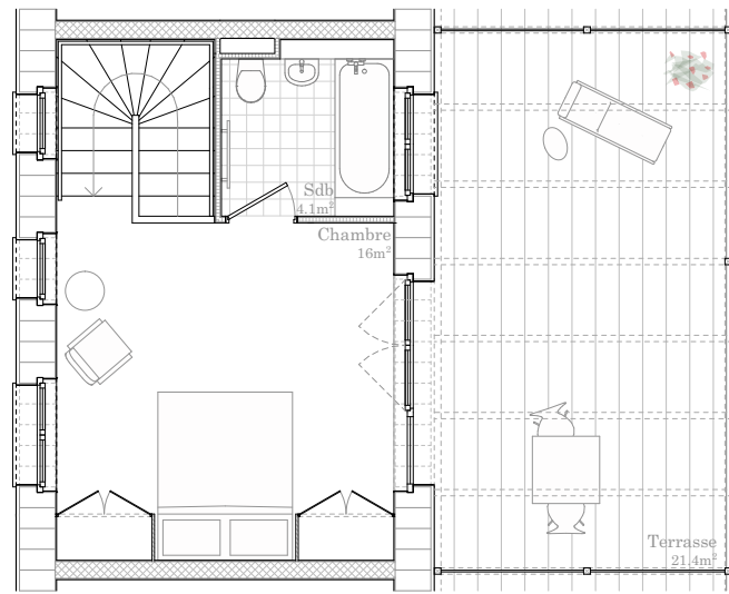
2e étage - Variante 1
