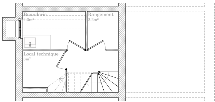
Sous-sol
