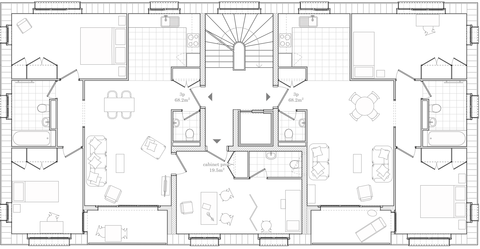
Étage type - Variante 1
