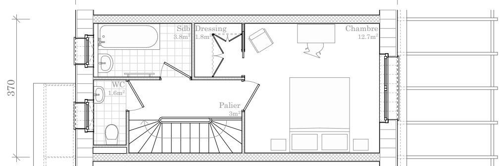
1er étage
