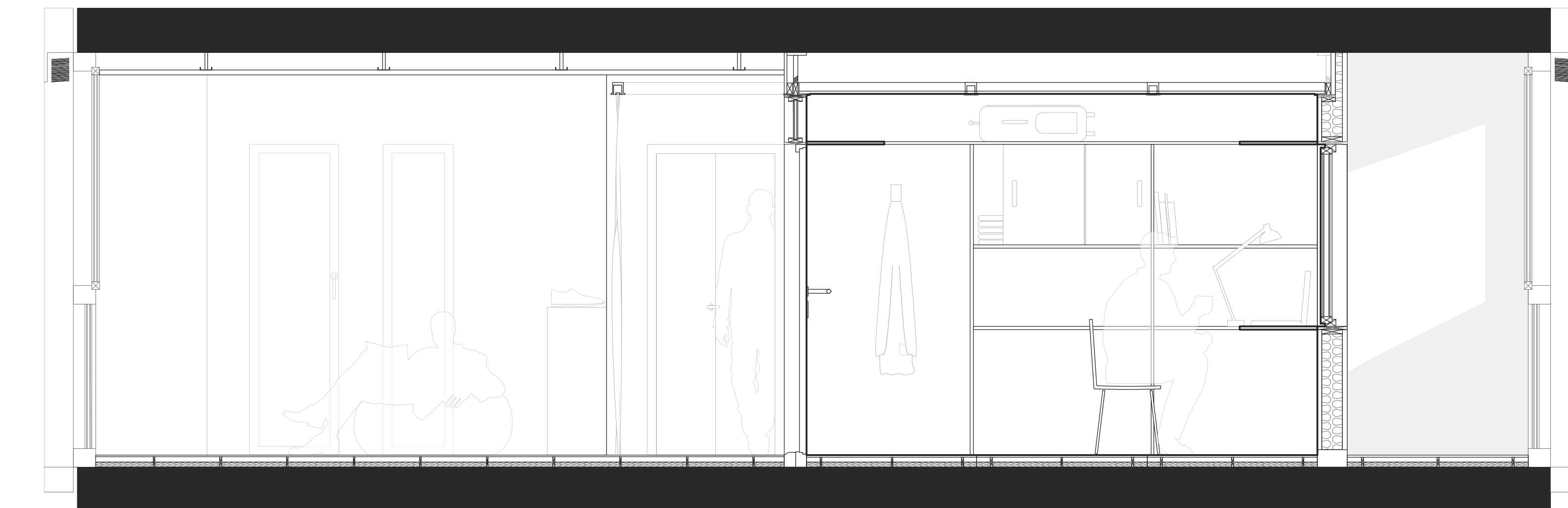
COUPE FOYER TATTES 1_25
