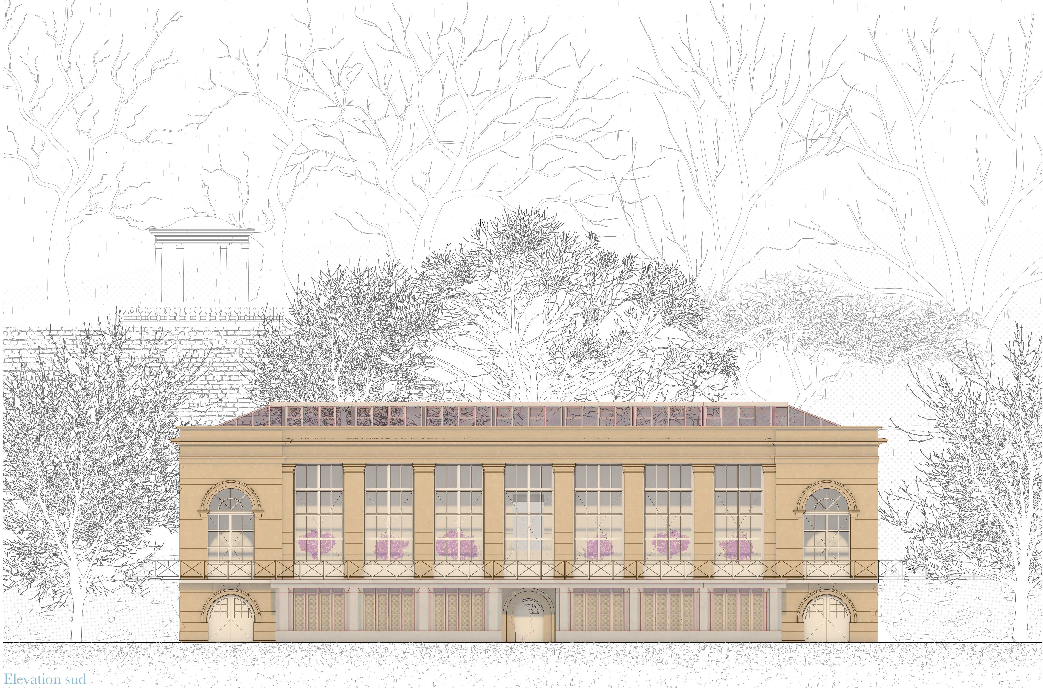
Elevation sud
