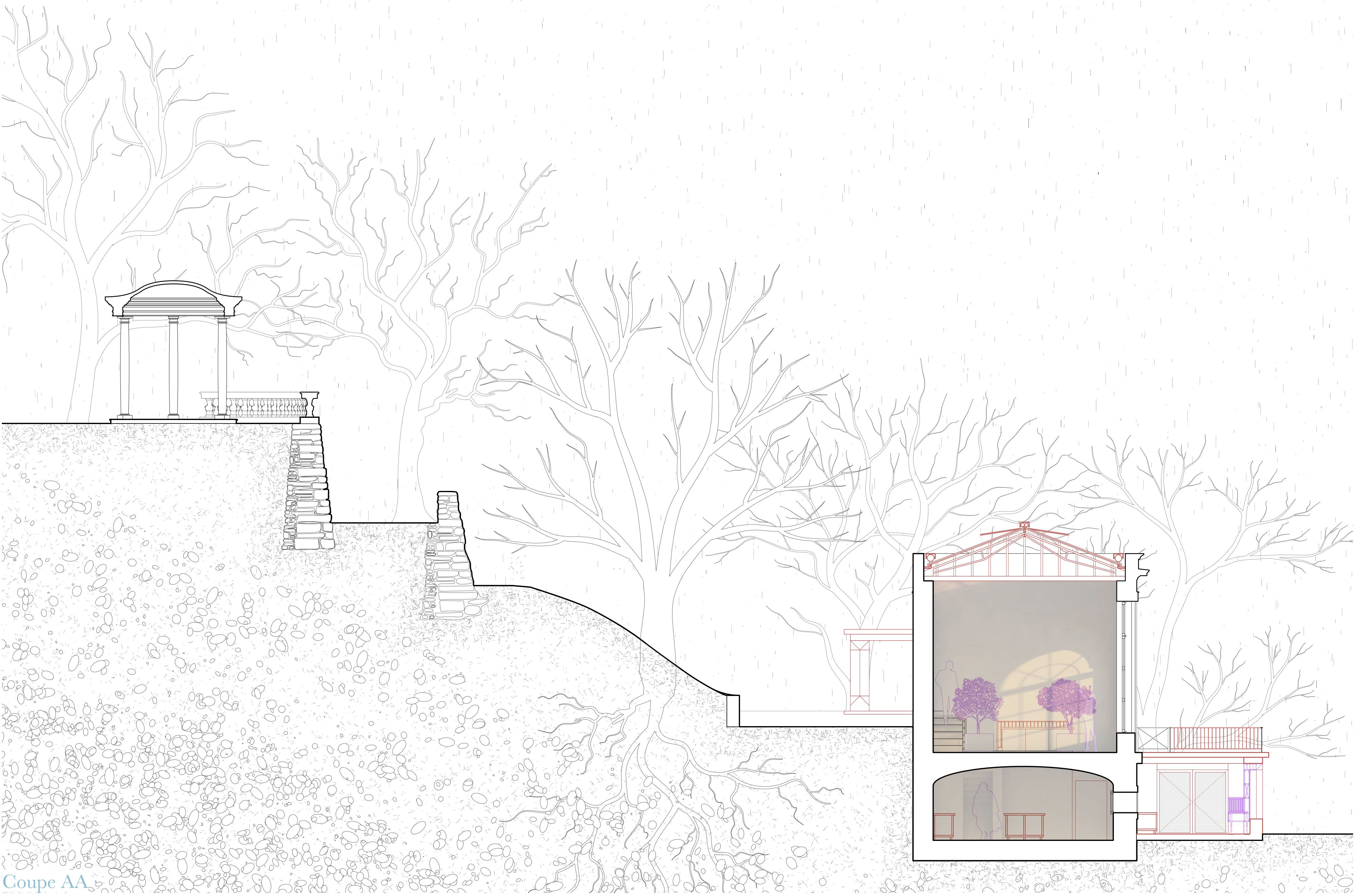
Coupe AA
