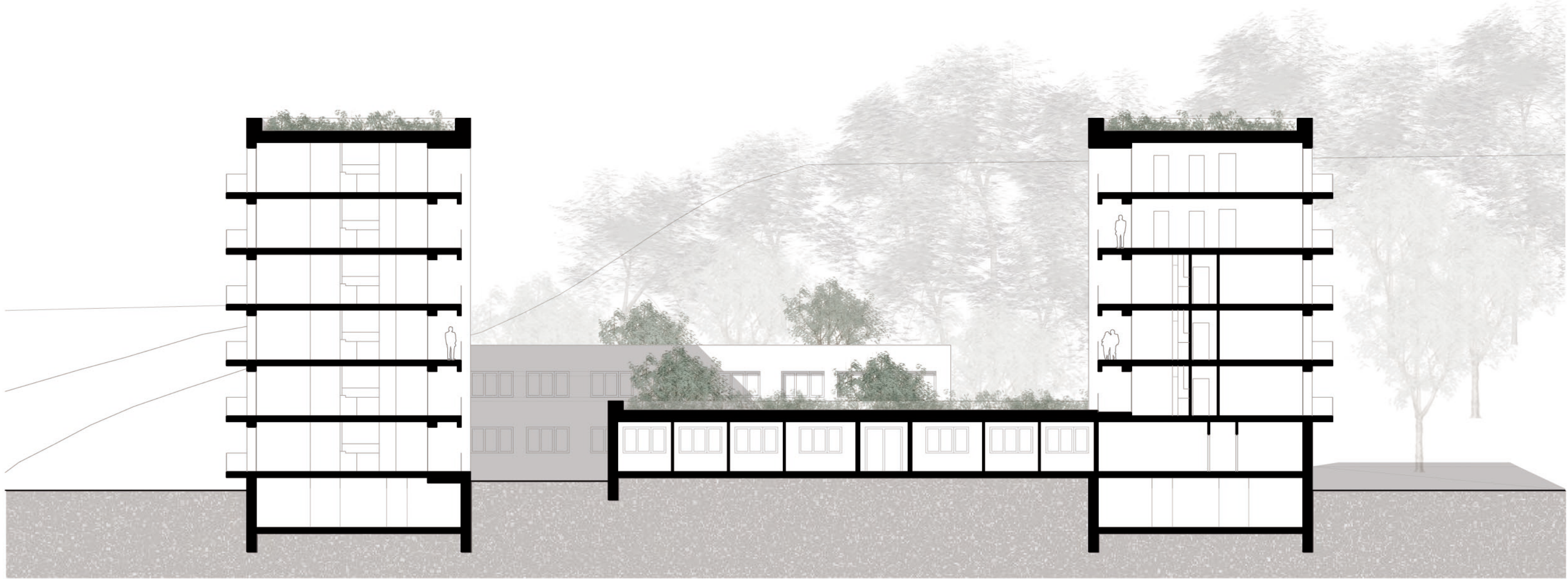
Coupe A 1/200
