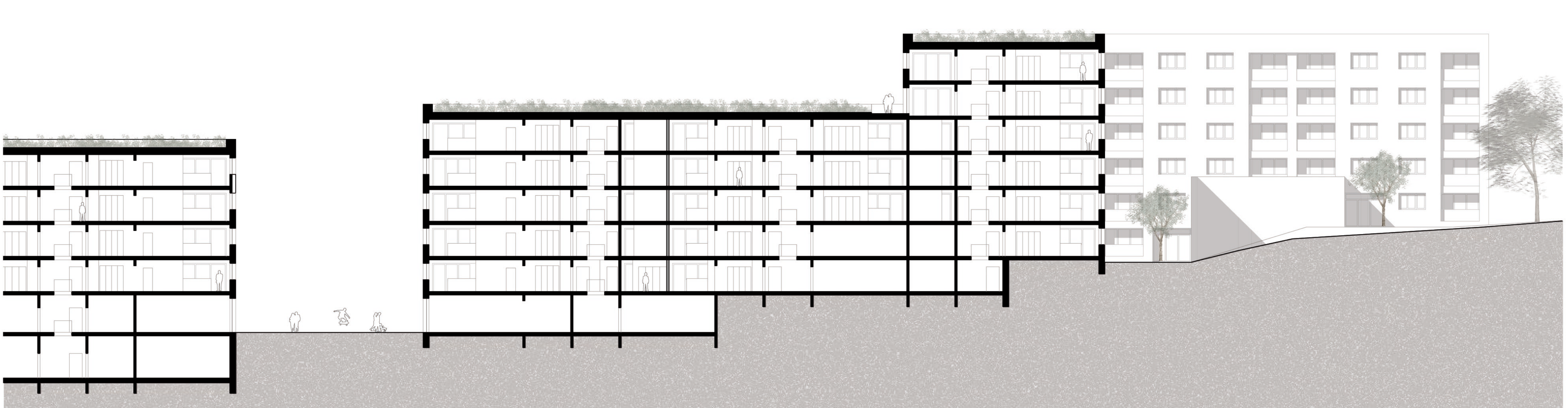
Coupe D 1/200
