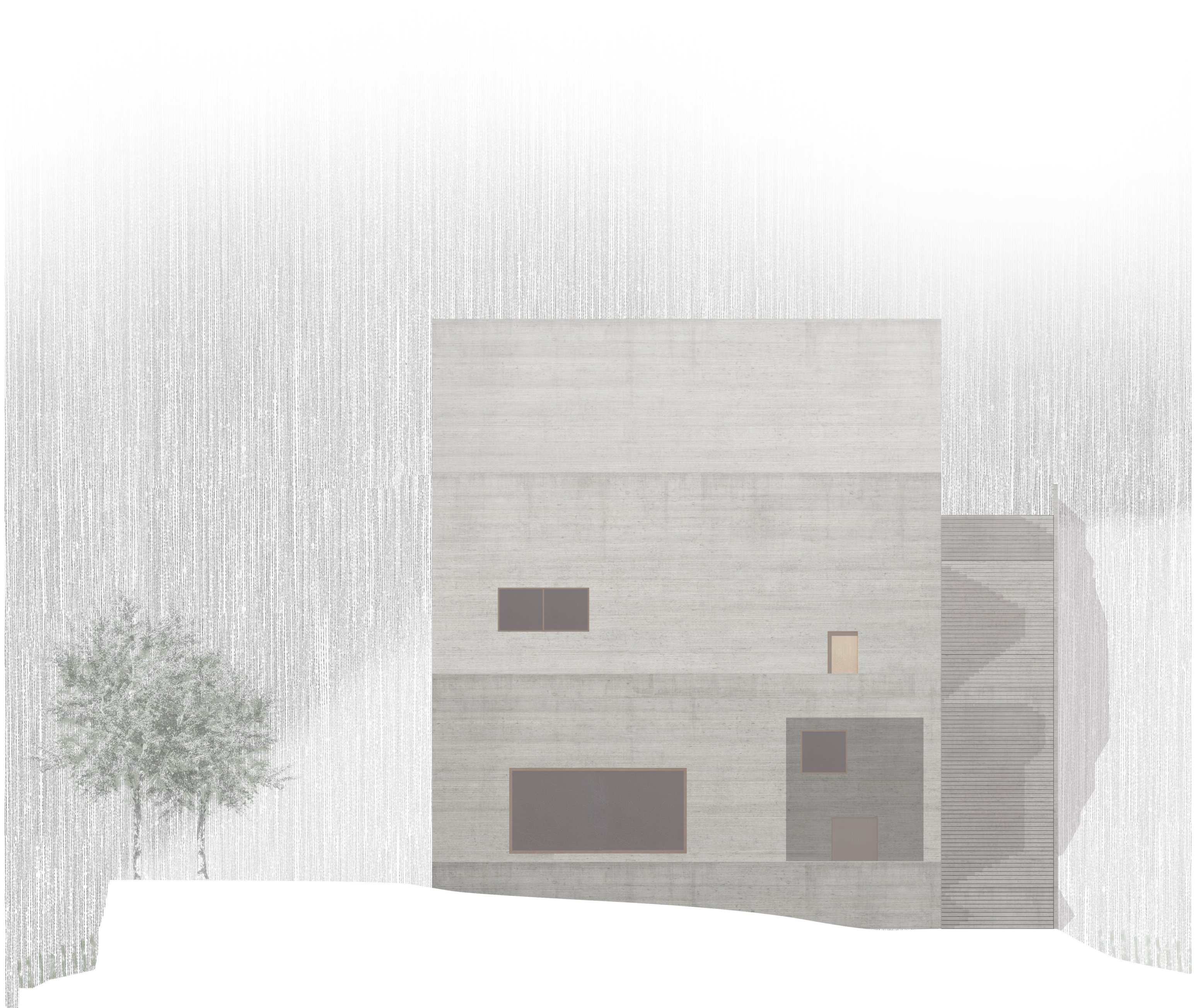
Élévation Sud-Est | 1:100
