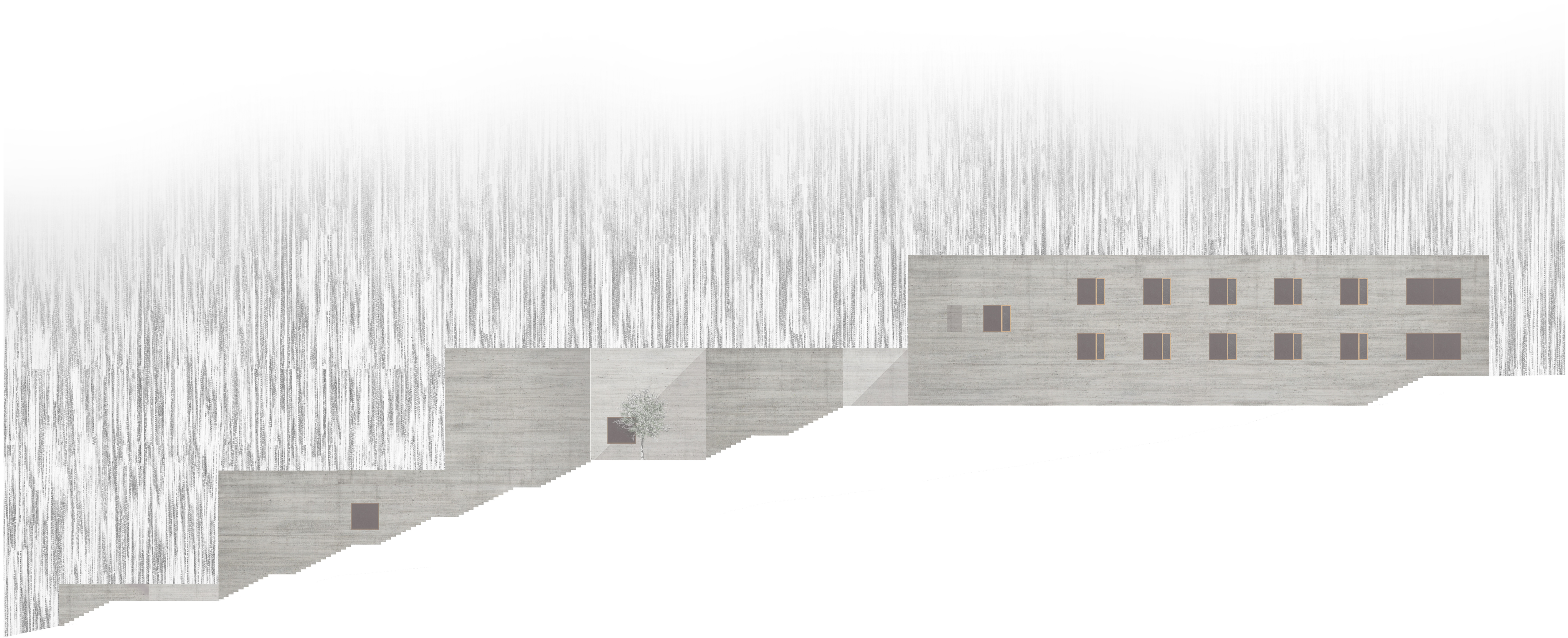
Élévation Nord-Est | 1:100
