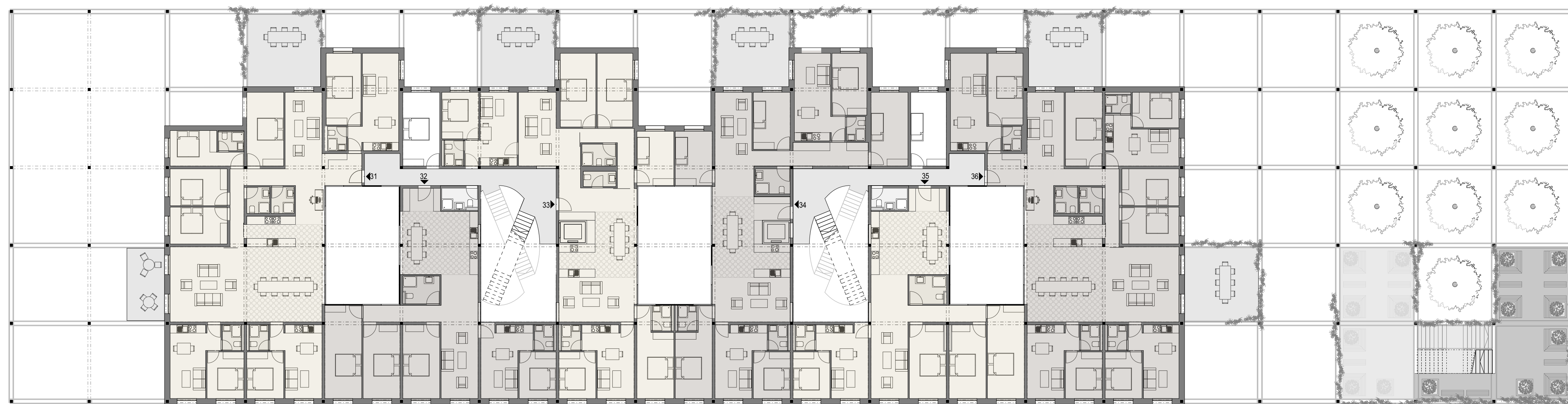
Étage 3 1: 200
