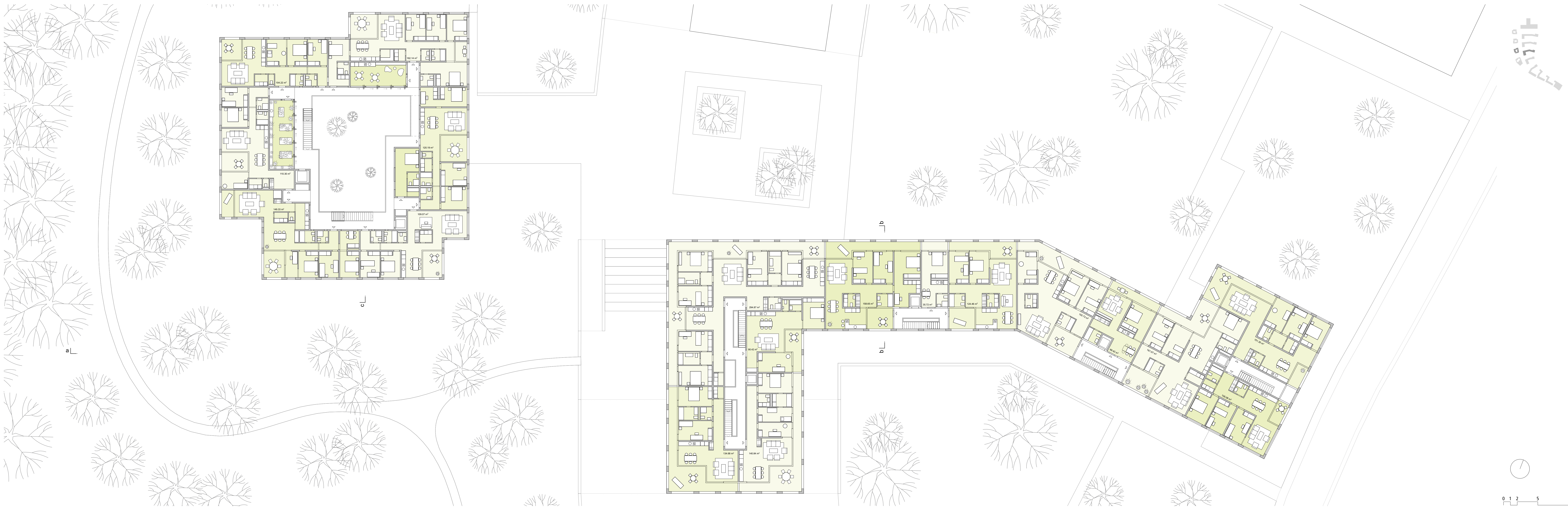
Plan d'étage type - 1:200
