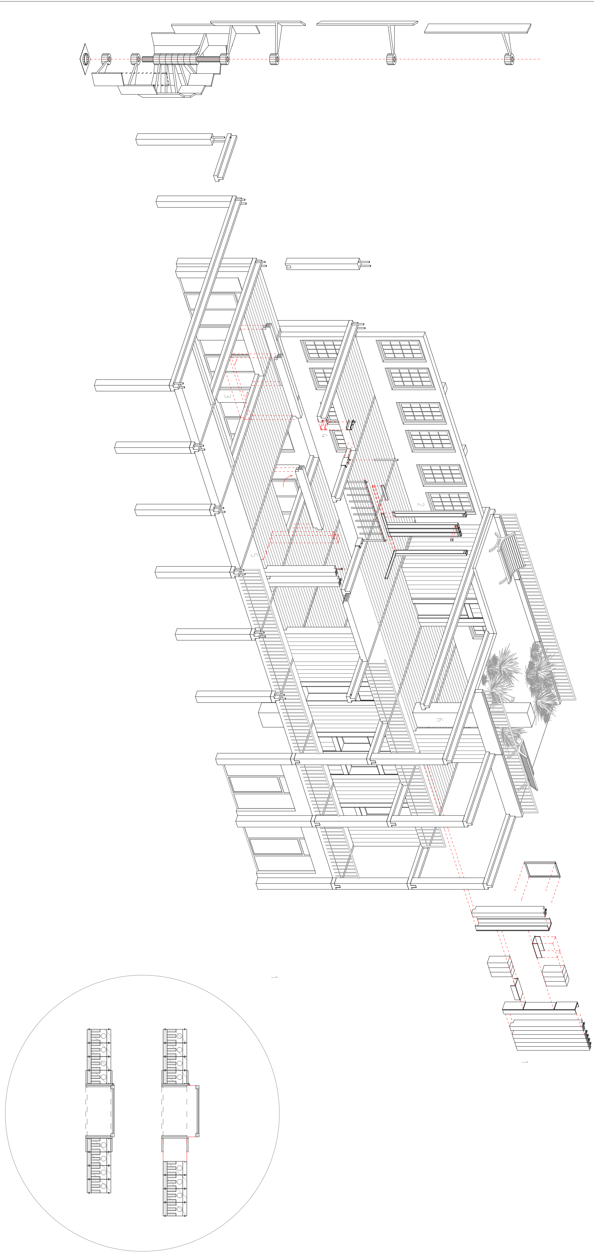
AXONOMÉTRIE D'ASSEMBLAGE
