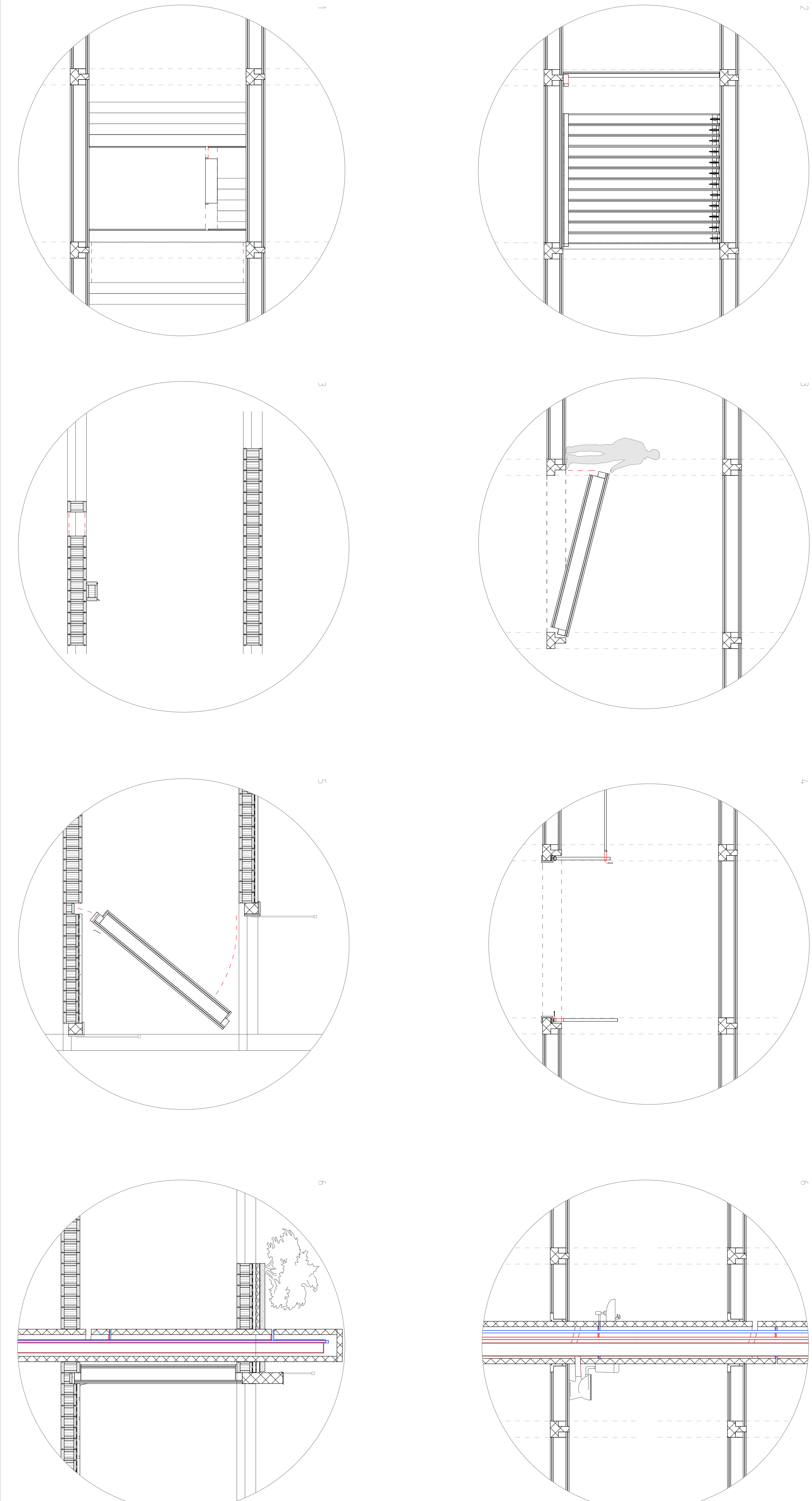
DÉTAILS D'ASSEMBLAGE
