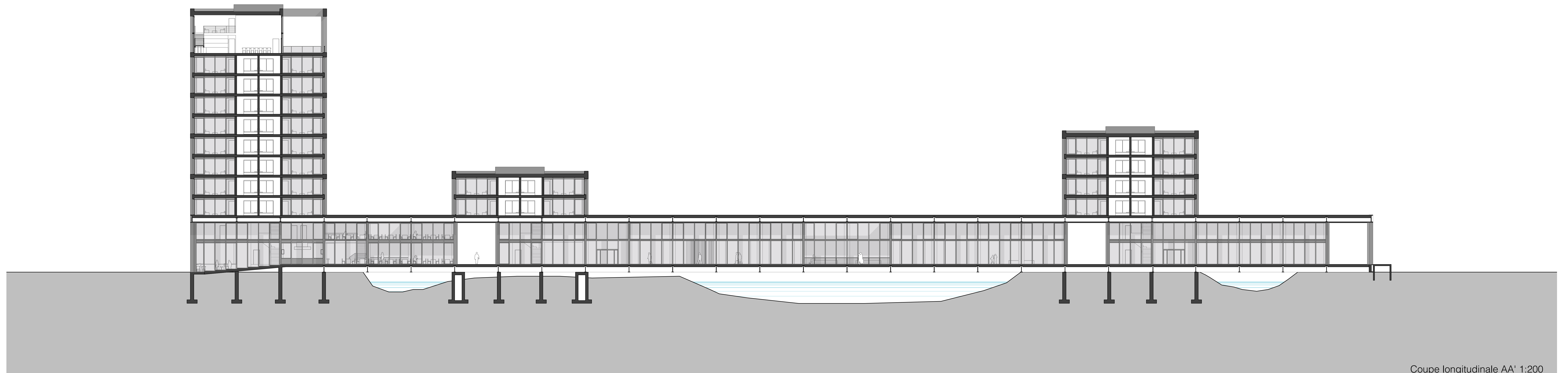
Coupe longitudinale AA' 1:200
