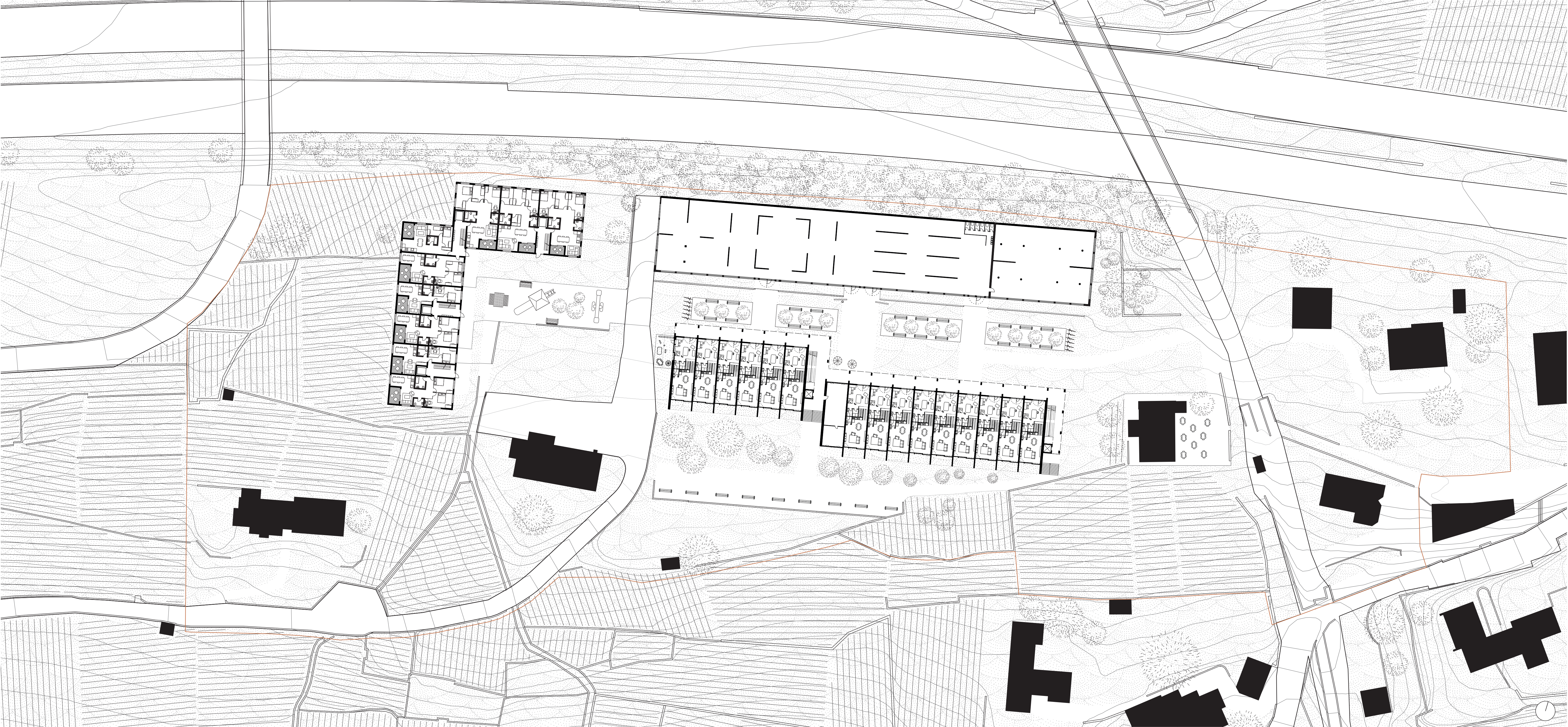
Plan des rez-de-chaussée 1:500
