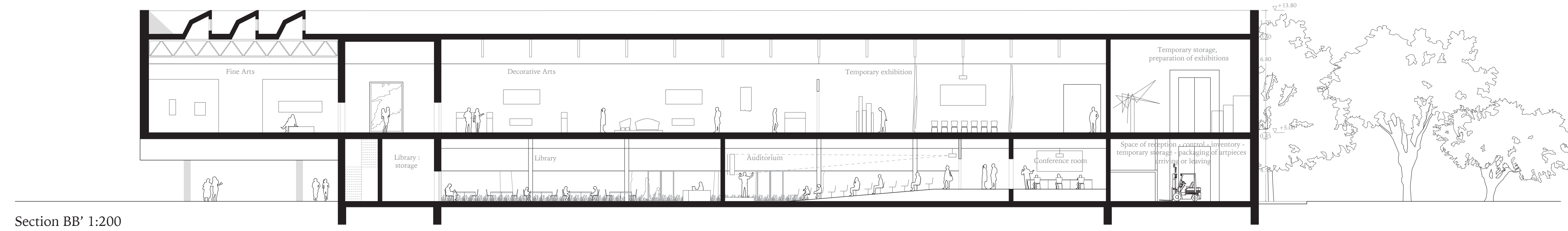
Section BB' 1:200
